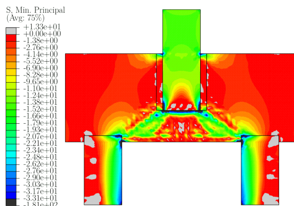
Figura 3.57 – Bielas de compressão do modelo EMB_L (MPa)
