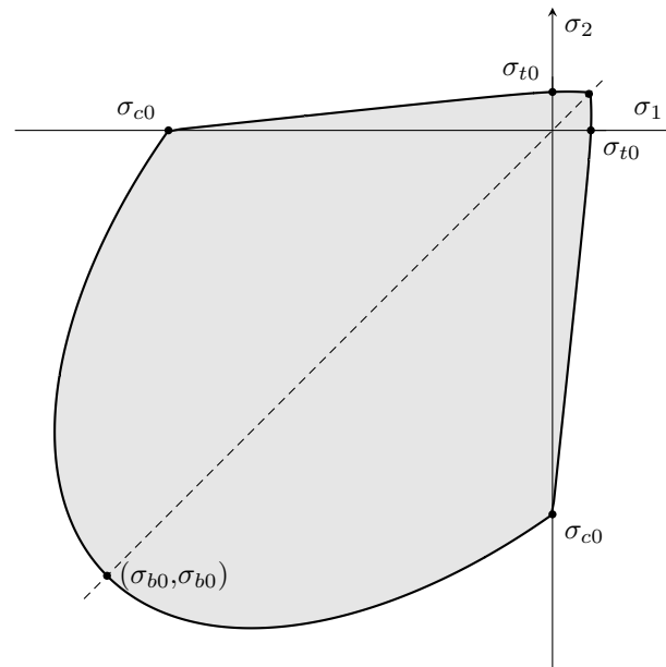
Figura 3.13 – Superfície de escoamento do CDP no estado plano de tensões
