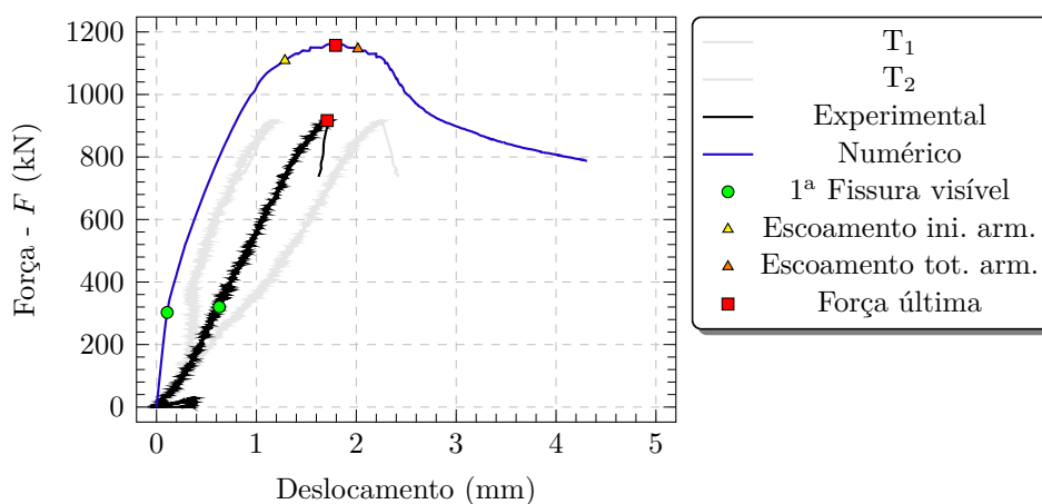
Figura 3.68 – Força-deslocamento do modelo EXT_C
