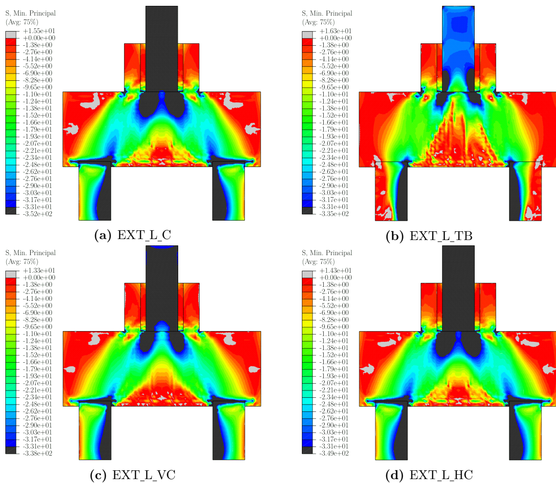
Figura 4.6 – Bielas de compressão dos blocos com cálice externo de interface lisa (MPa)
