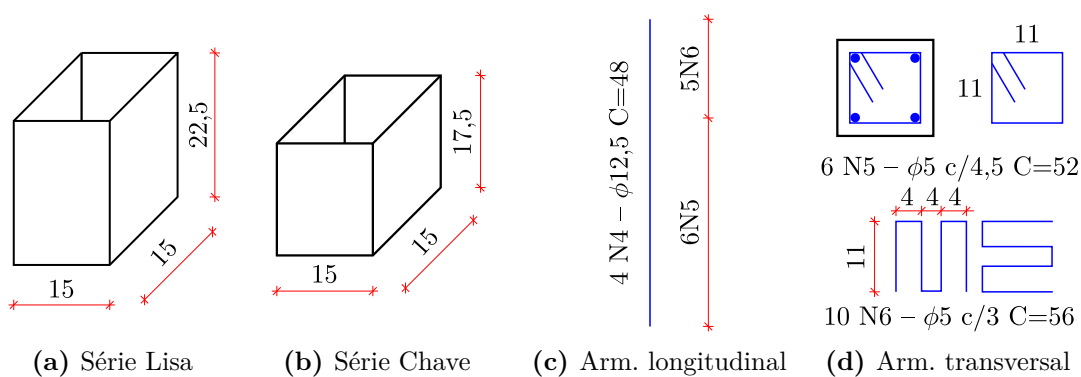
Figura A.1 – Propriedades geométricas dos pilares de concreto pré-moldado (cm)
