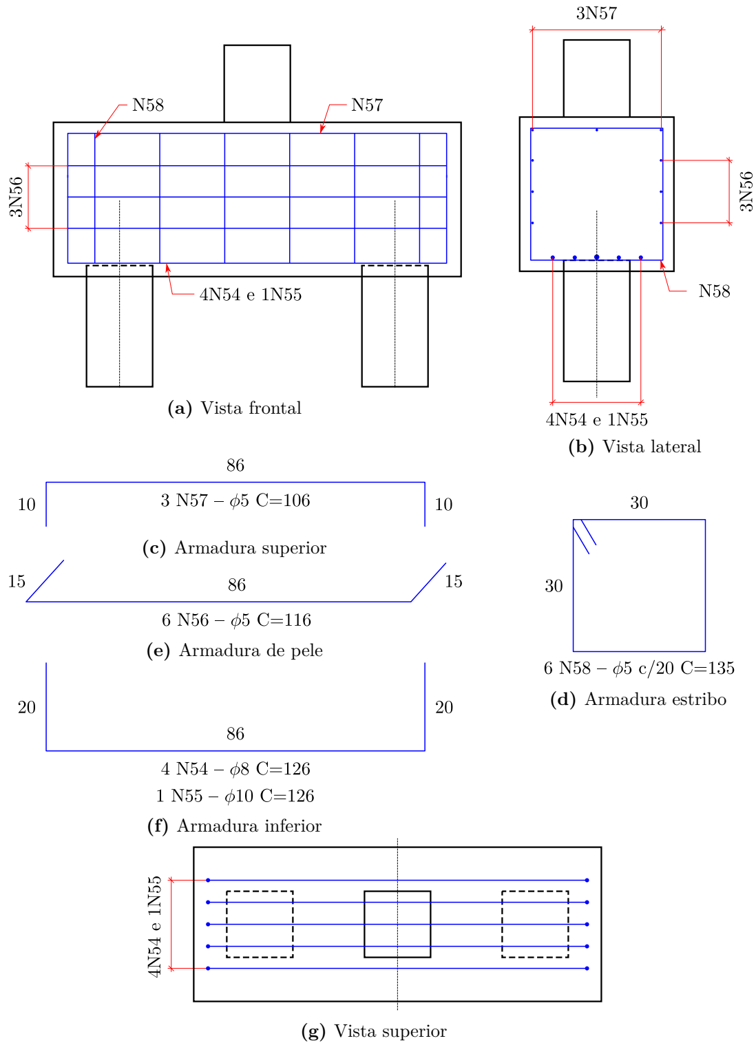
Figura A.5 – Detalhamento do bloco monolítico da série lisa (cm)
