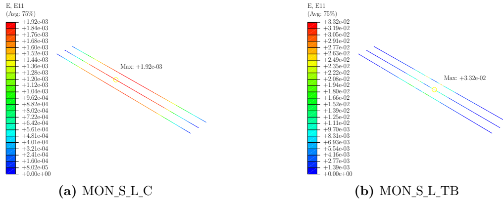
Figura 4.4 – Distribuição de deformações nos tirantes principais dos blocos monolíticos de referência da série lisa
