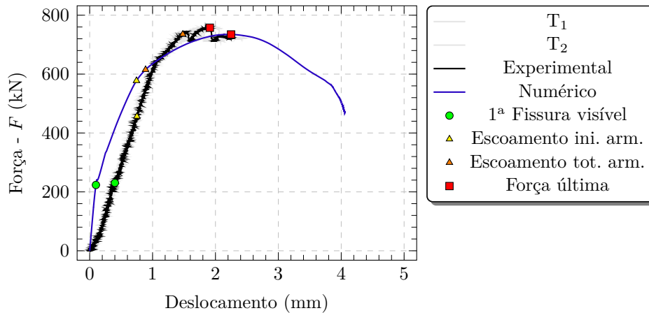
Figura 3.40 – Força-deslocamento do modelo MON_S_L
