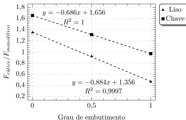
Figura 4.57 – Influência do grau de embutimento
