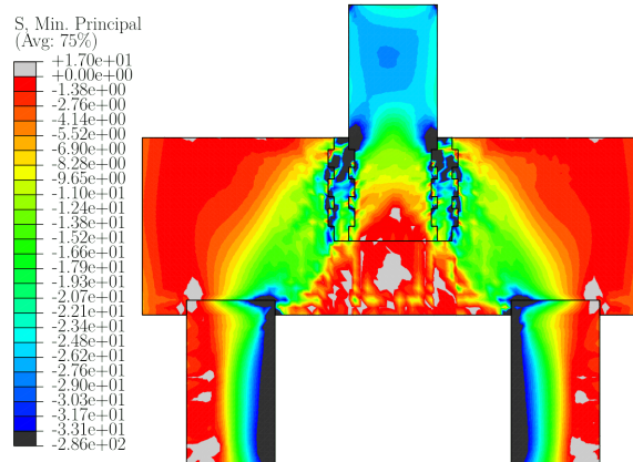
Figura 3.81 – Bielas de compressão do modelo EMB_C (MPa)
