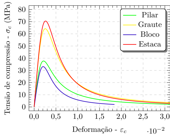
Figura 3.25 – Diagrama tensão-deformação à compressão nos concretos
