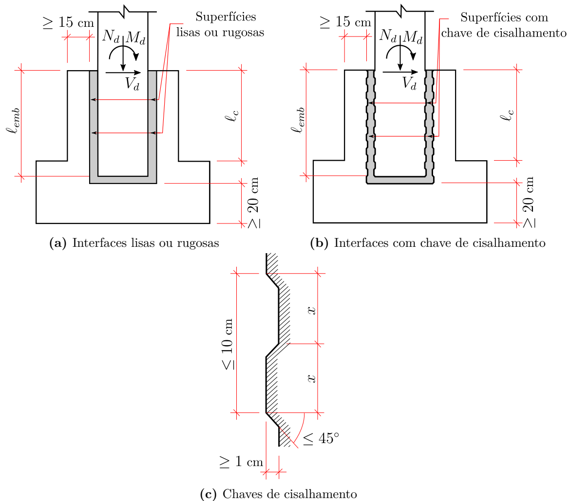
Figura 2.36 – Transferência dos esforços nas paredes do colarinho dos cálices de interfaces lisas ou rugosas
