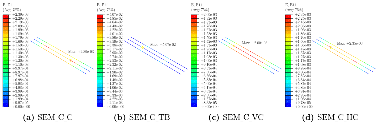
Figura 4.44 – Distribuição de deformações nos tirantes principais dos blocos com cálice semiembutido de interface com chave de cisalhamento
