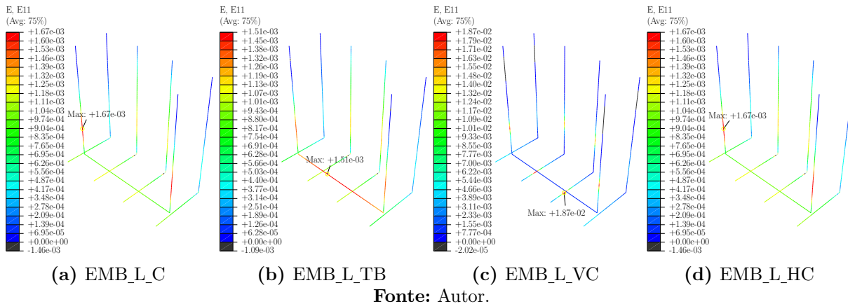
Figura 4.26 – Distribuição de deformações nas armaduras verticais dos cálices embutidos liso
