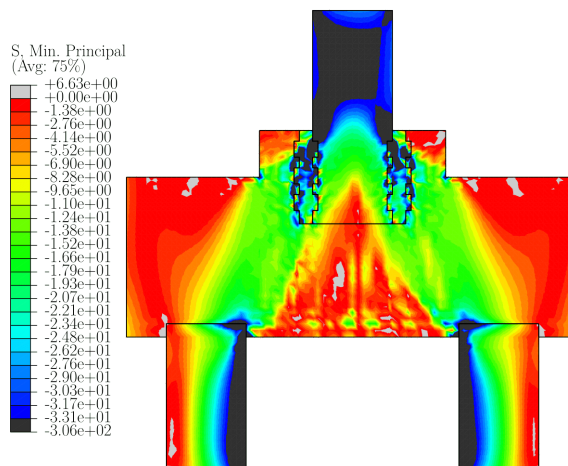
Figura 3.73 – Bielas de compressão do modelo SEM_C (MPa)
