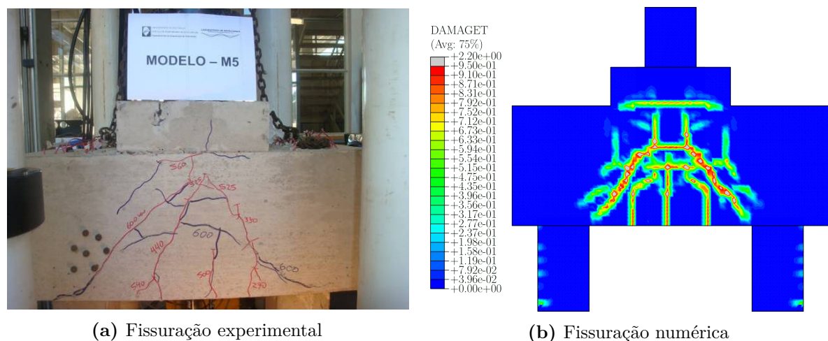
Figura 3.55 – Panorama de fissuração do modelo SEM_AC_L
