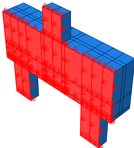
Figura 3.33 – Condição de contorno de simetria
