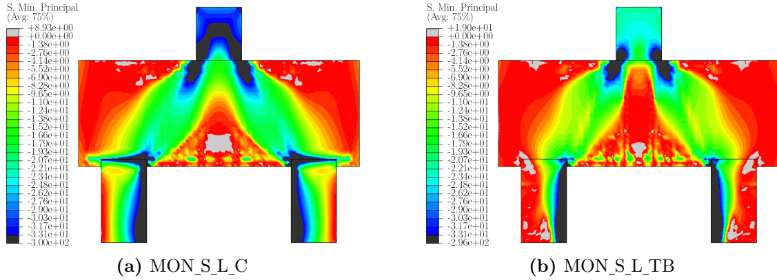
Figura 4.2 – Bielas de compressão dos blocos monolíticos de referência da série lisa (MPa)
