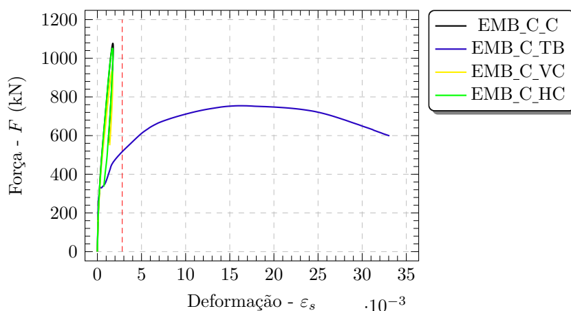
Figura 4.51 – Curvas força-deformação nos tirantes principais dos blocos com cálice embutido de interface com chave de cisalhamento
