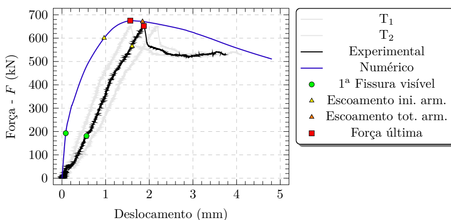
Figura 3.80 – Força-deslocamento do modelo EMB_C
