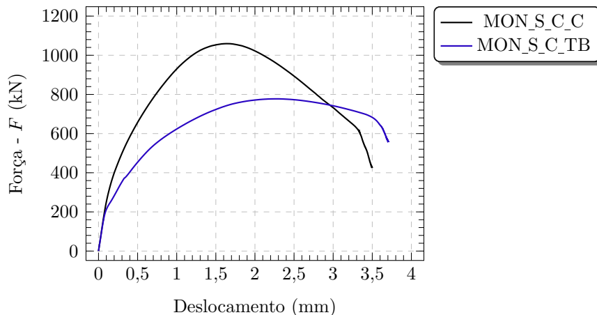
Figura 4.29 – Curvas força-deslocamento dos blocos monolíticos de referência da série com chave de cisalhamento
