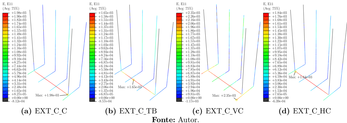
Figura 4.38 – Distribuição de deformações nas armaduras verticais dos cálices externos de interface com chave de cisalhamento
