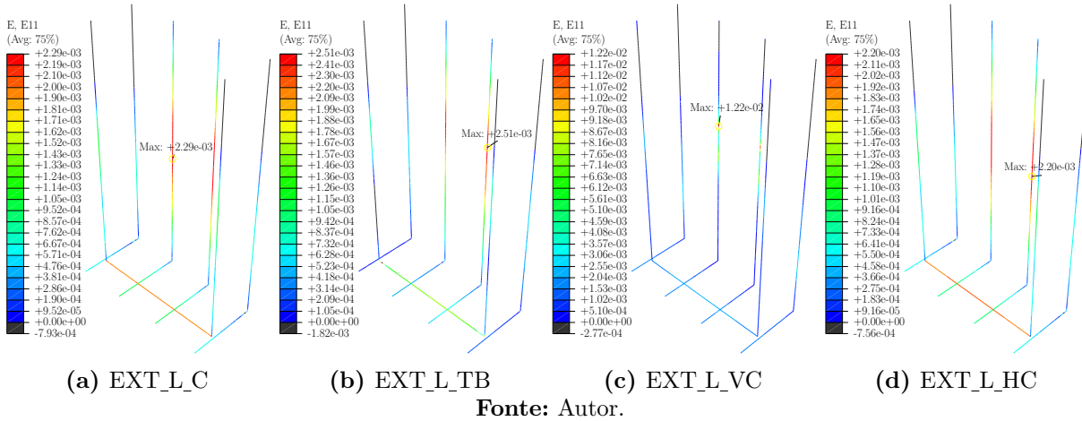
Figura 4.10 – Distribuição de deformações nas armaduras verticais dos cálices externos de interface lisa
