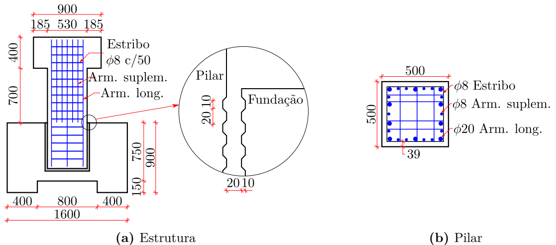
Figura 2.27 – Detalhes geométricos e de armação do modelo de cálice embutido (un: mm)
