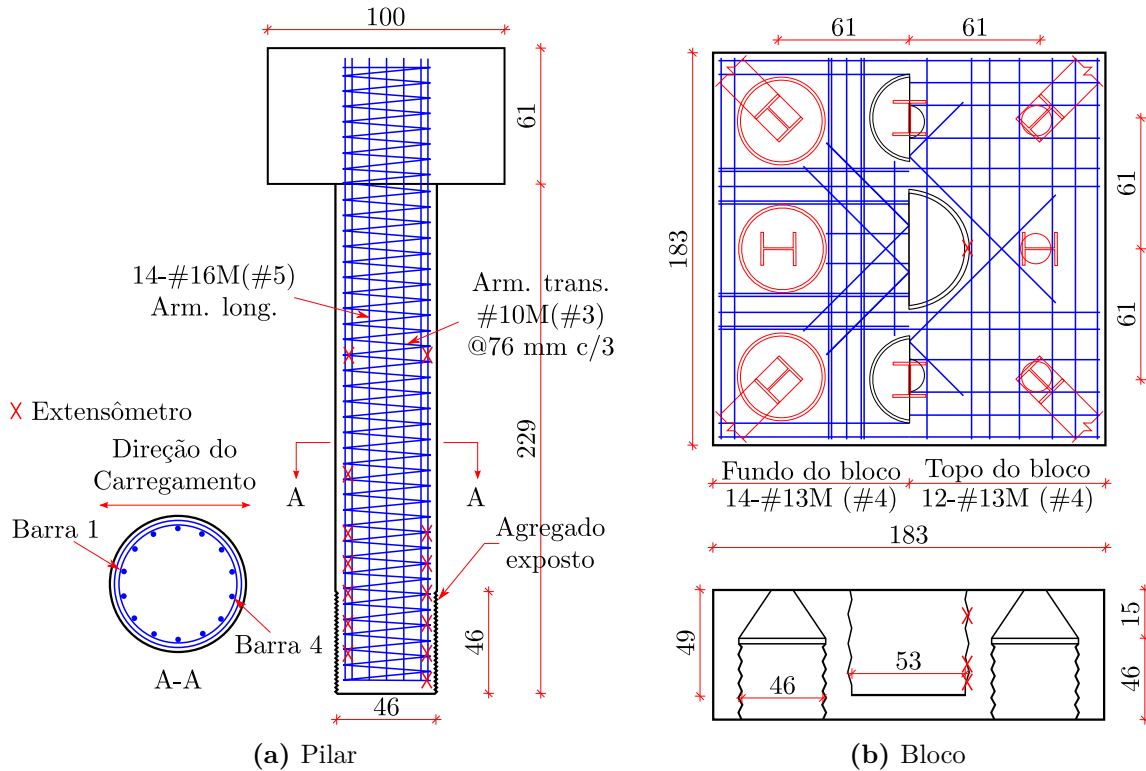
Figura 2.24 – Dimensões e detalhes estruturais do modelo ensaiado (un: cm)
