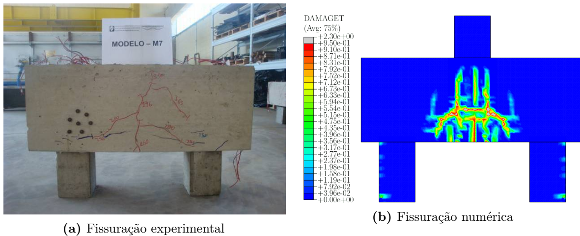
Figura 3.63 – Panorama de fissuração do modelo EMB_AC_L
