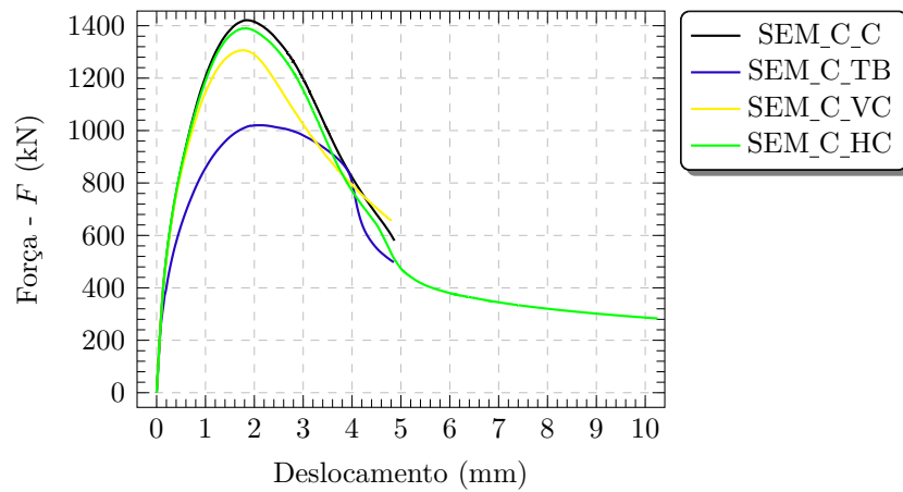
Figura 4.41 – Curvas força-deslocamento dos blocos com cálice semiembutido de interface com chave de cisalhamento
