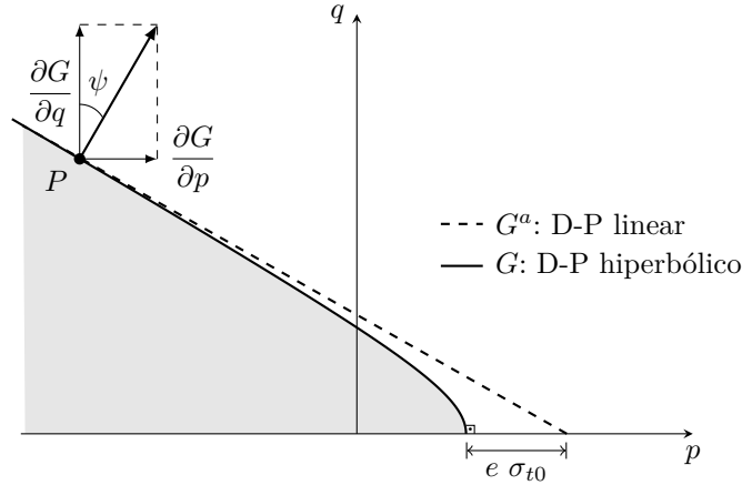
Figura 3.17 – Função potencial plástico G no plano p - q
