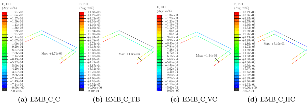
Figura 4.56 – Distribuição de deformações nas armaduras horizontais dos cálices embutidos de interface com chave de cisalhamento
