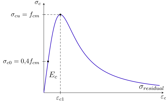
Figura 3.24 – Modelo do diagrama tensão-deformação à compressão no concreto
