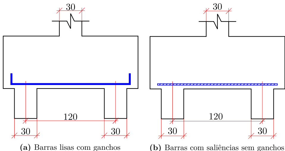
Figura 2.8 – Bloco sobre duas estacas de Blevot e Frémy (1967)
