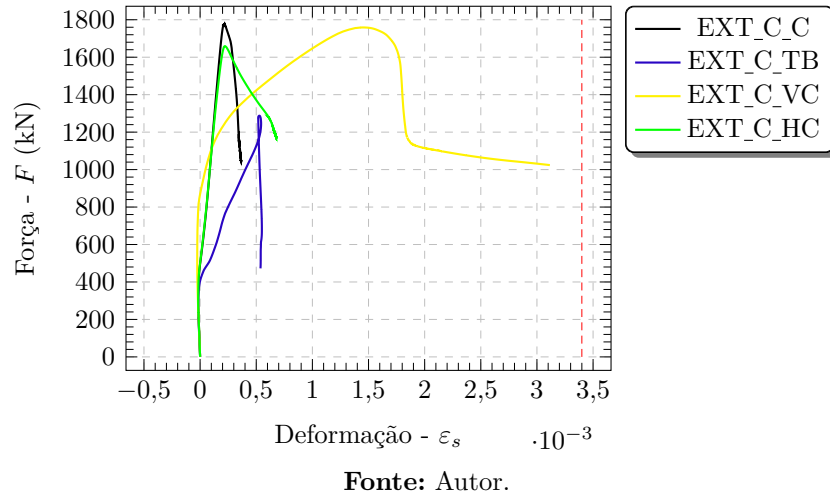
Figura 4.37 – Curvas força-deformação nas armaduras verticais dos cálices externos de interface com chave de cisalhamento
