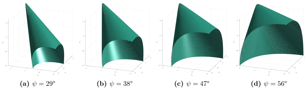
Figura 3.20 – Influência do parâmetro \psi na superfície do potencial plástico do CDP no espaço tridimensional de tensões
