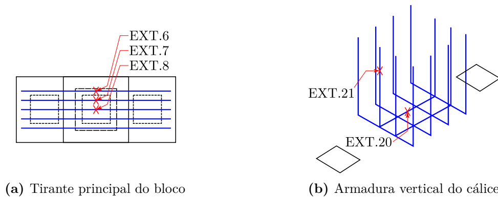
Figura 3.3 – Posição dos extensômetros nas armaduras do bloco e do cálice de fundação
