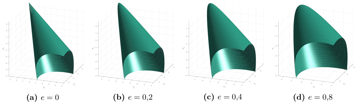
Figura 3.18 – Influência da excentricidade e na superfície do potencial plástico do CDP no espaço tridimensional de tensões
