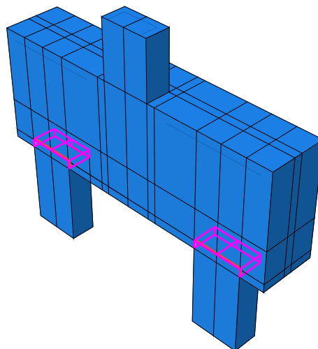
Figura 3.32 – Ligação do bloco de fundação com as estacas
