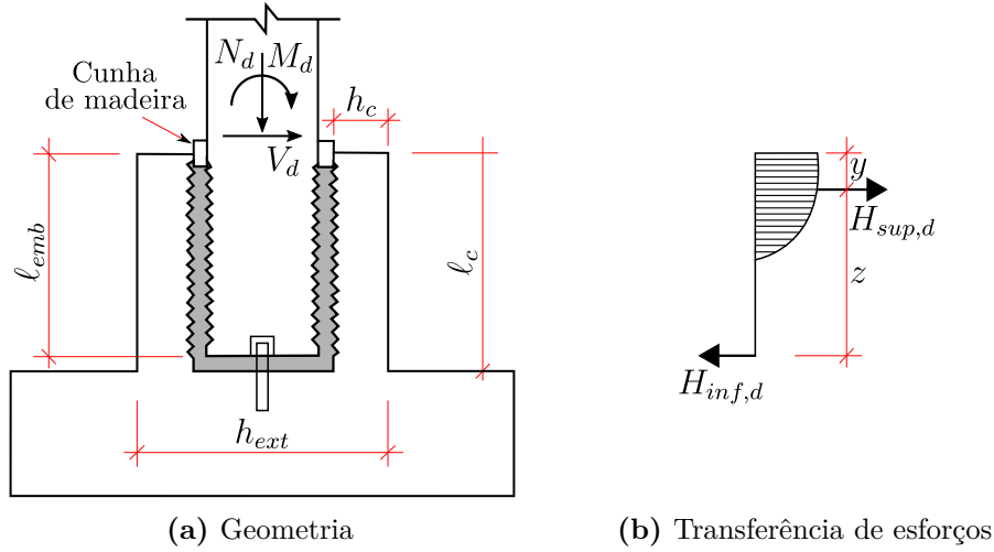
Figura 2.14 – Modelo de cálice rugoso de Leonhardt e Mönnig (1978)
