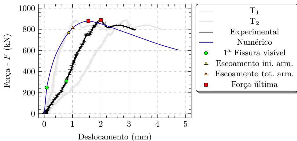
Figura 3.72 – Força-deslocamento do modelo SEM_C
