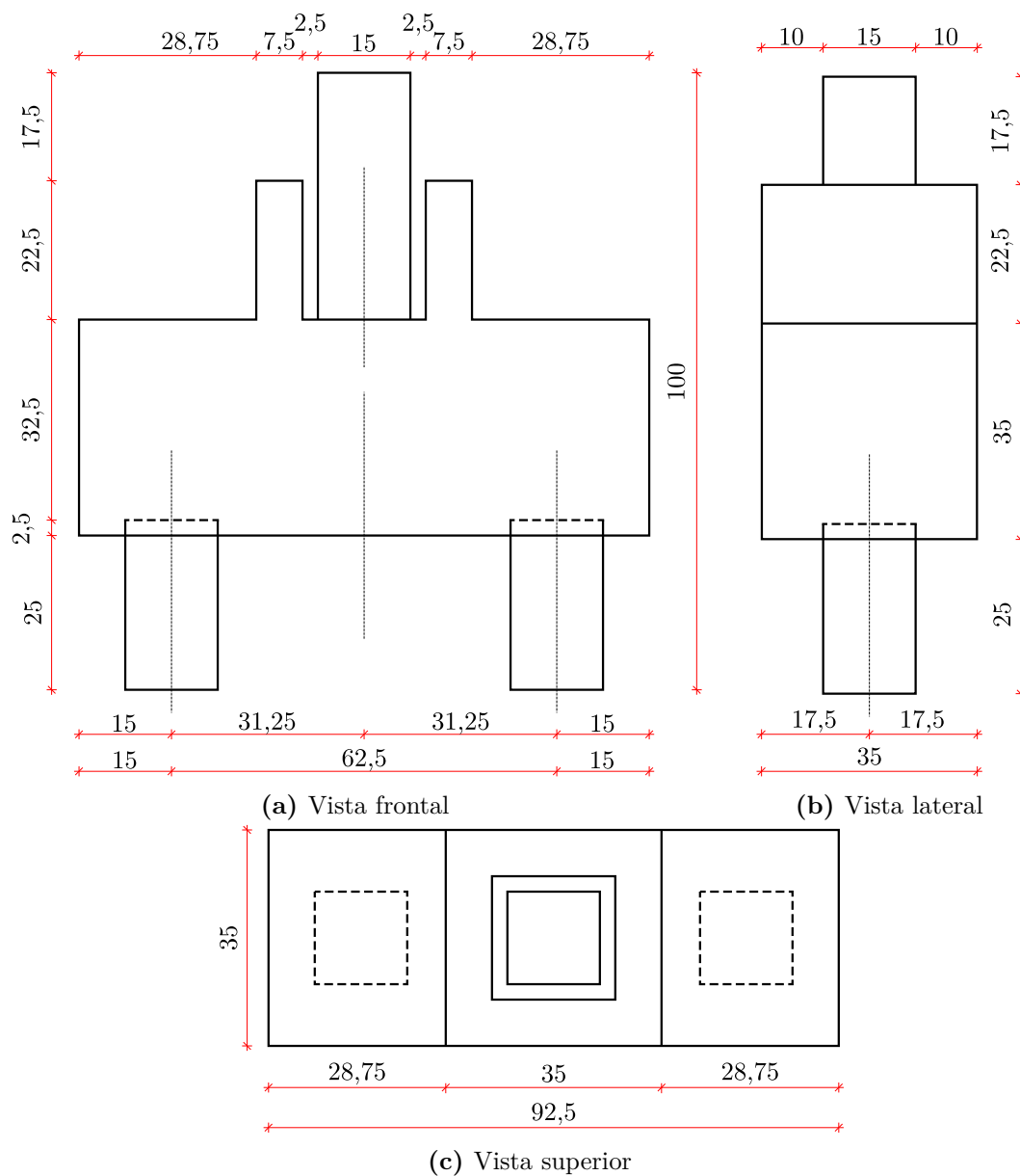
Figura A.6 – Propriedades geométricas do bloco com cálice externo da série lisa (cm)
