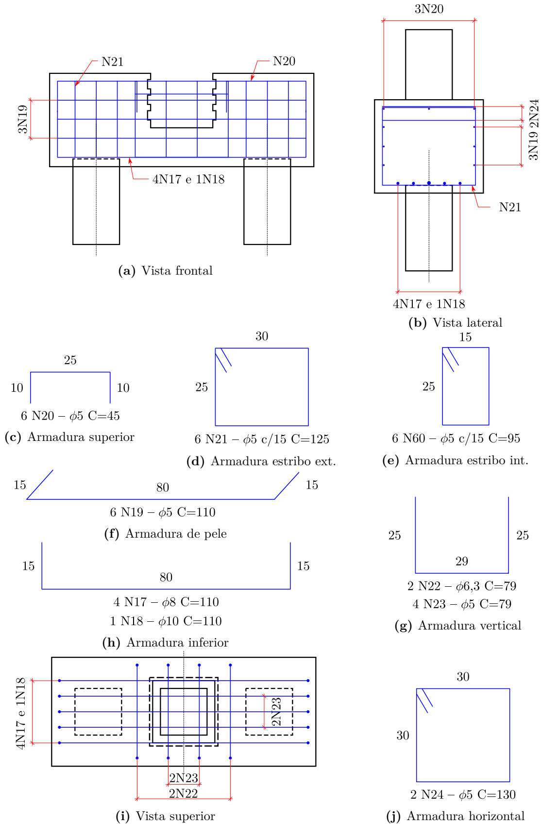
Figura A.19 – Detalhamento do bloco embutido da série com chave de cisalhamento (cm)
