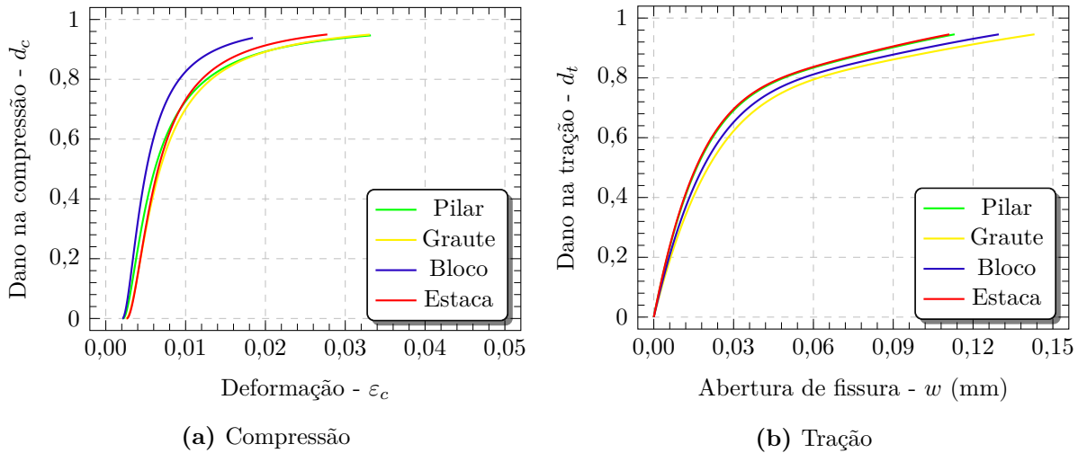
Figura 3.28 – Modelo de dano
