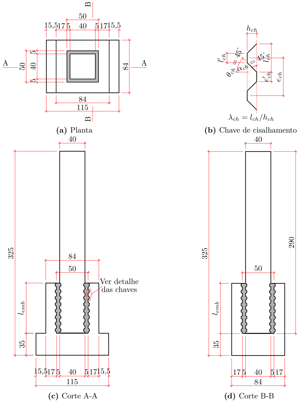
Figura 2.32 – Modelo proposto ensaiado por Canha (2004) (un: cm)
