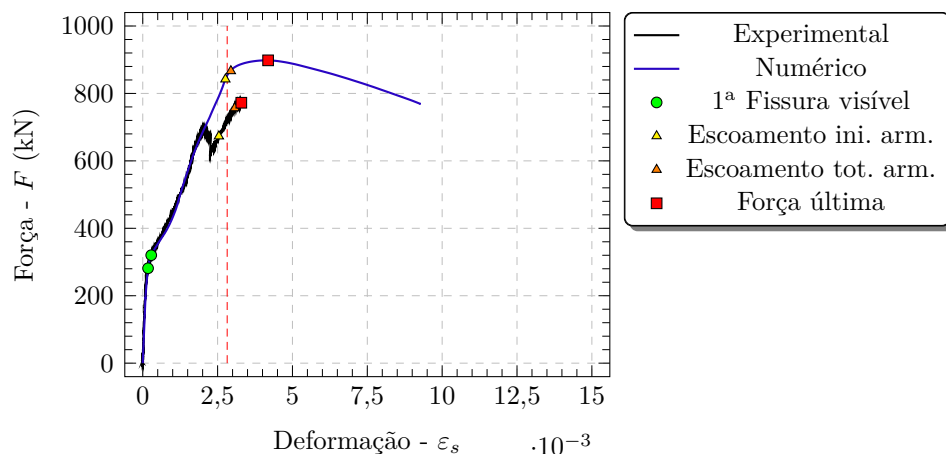
Figura 3.46 – Força-deformação tirante do bloco do modelo EXT_L
