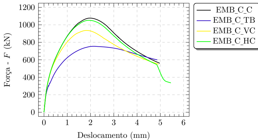
Figura 4.49 – Curvas força-deslocamento dos blocos com cálice embutido de interface com chave de cisalhamento
