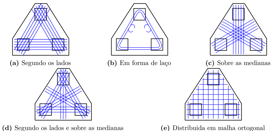
Figura 2.9 – Arranjo de armaduras em blocos de três estacas de Blevot e Frémy (1967)
