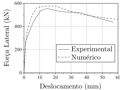
Figura 2.28 – Curva força lateral-deslocamento
