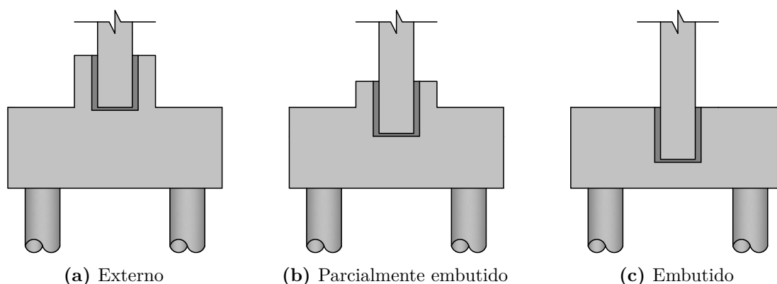
Figura 1.1 – Classificações do cálice de fundação de acordo com o grau embutimento
