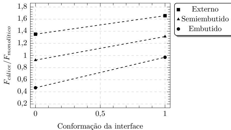
Figura 4.58 – Conformação da interface
