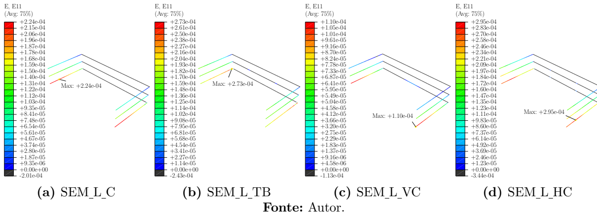
Figura 4.20 – Distribuição de deformações nas armaduras horizontais dos cálices semiembutidos de interface lisa
