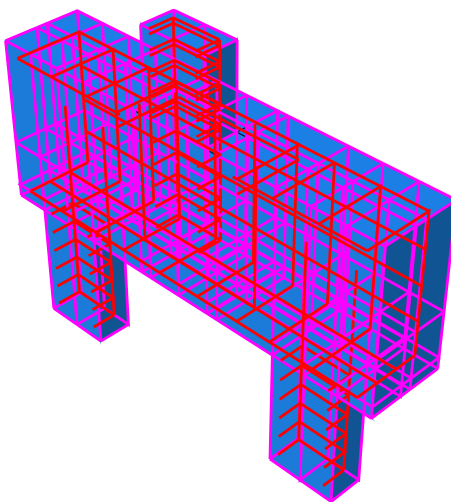
Figura 3.29 – Armaduras embutidas nos elementos de concreto
