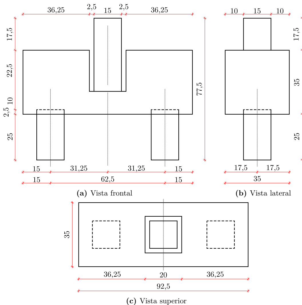
Figura A.10 – Propriedades geométricas do bloco com cálice embutido liso (cm)
