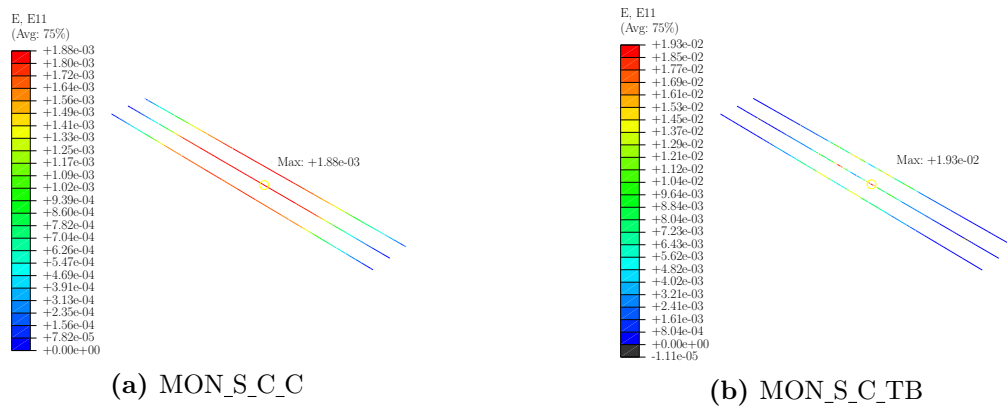
Figura 4.32 – Distribuição de deformações nos tirantes principais dos blocos monolíticos de referência da série com chave de cisalhamento
