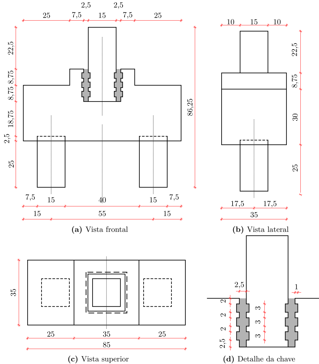
Figura A.16 – Propriedades geométricas do bloco com cálice semiembutido da série com chave de cisalhamento (cm)
