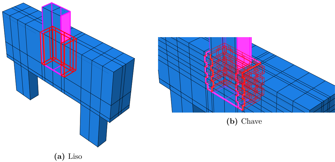
Figura 3.31 – Interação de contato entre o pilar-graute e o graute-bloco
