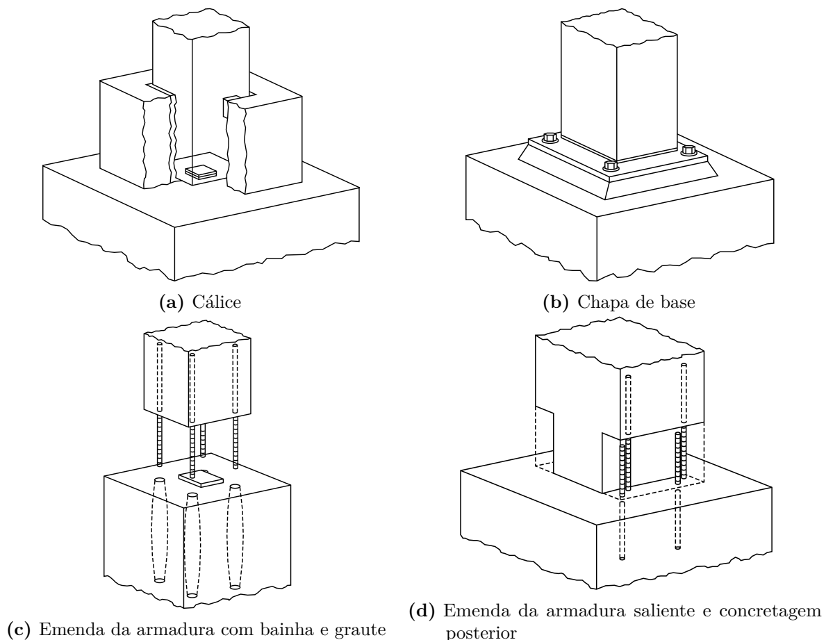
Figura 2.1 – Tipos de ligações pré-moldadas pilar-fundação
