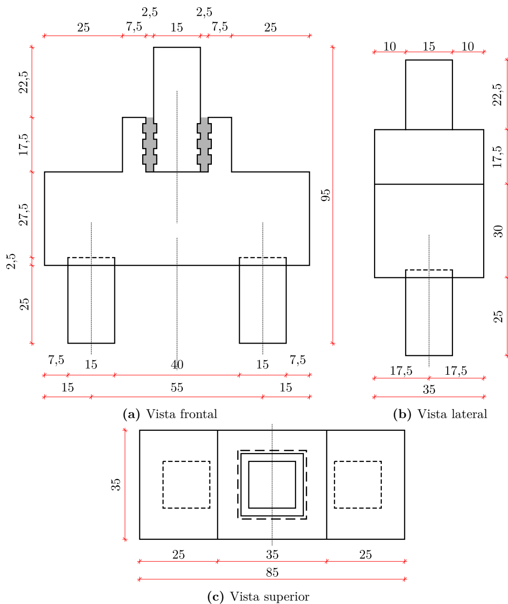
Figura A.14 – Propriedades geométricas do bloco com cálice externo da série com chave de cisalhamento (cm)
