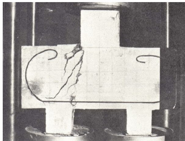
Figura 2.12 – Ruína do modelo ensaiado por Mautoni (1972)
