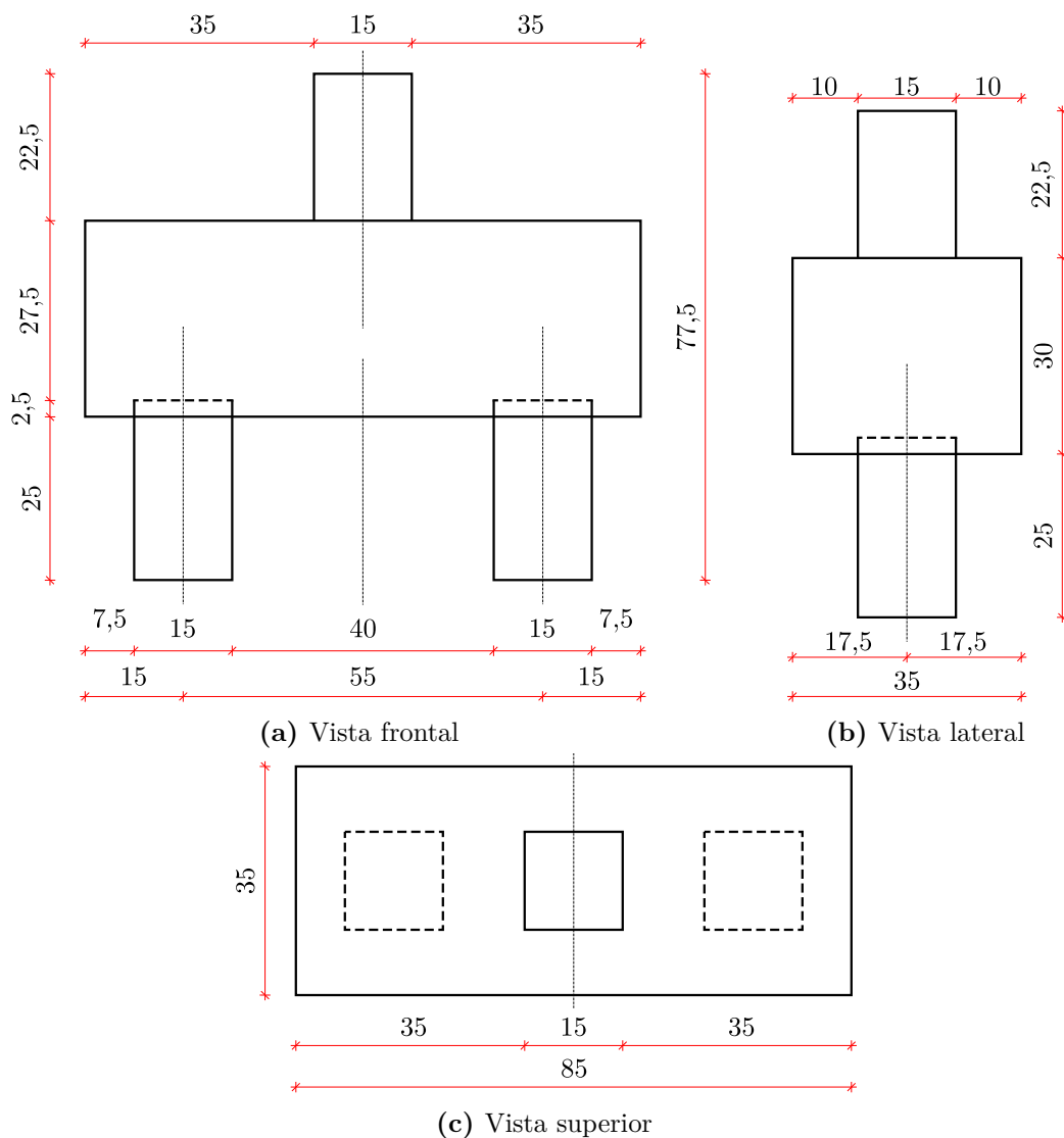
Figura A.12 – Propriedades geométricas do bloco monolítico da série com chave de cisalhamento (cm)
