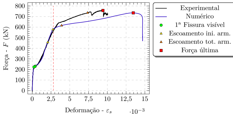
Figura 3.42 – Força-deformação tirante do bloco do modelo MON_S_L
