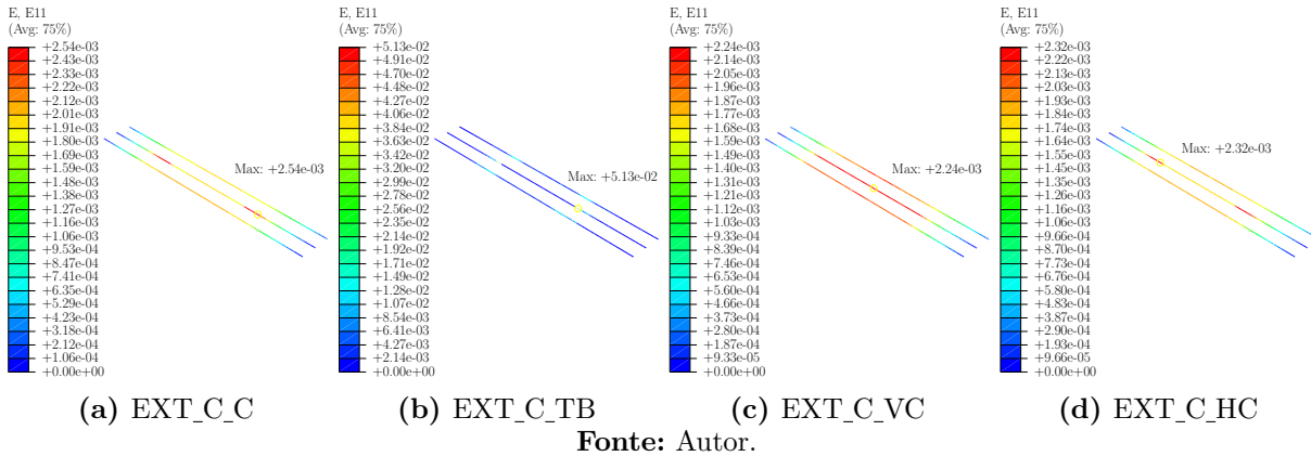
Figura 4.36 – Distribuição de deformações nos tirantes principais dos blocos com cálice externo de interface com chave de cisalhamento
