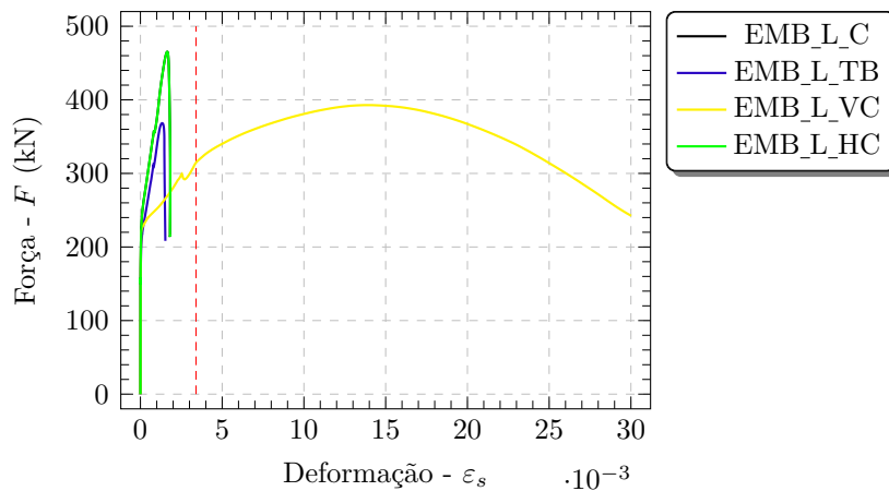
Figura 4.25 – Curvas força-deformação nas armaduras verticais dos cálices embutidos lisos
