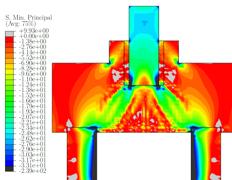
Figura 3.49 – Bielas de compressão do modelo SEM_L (MPa)
