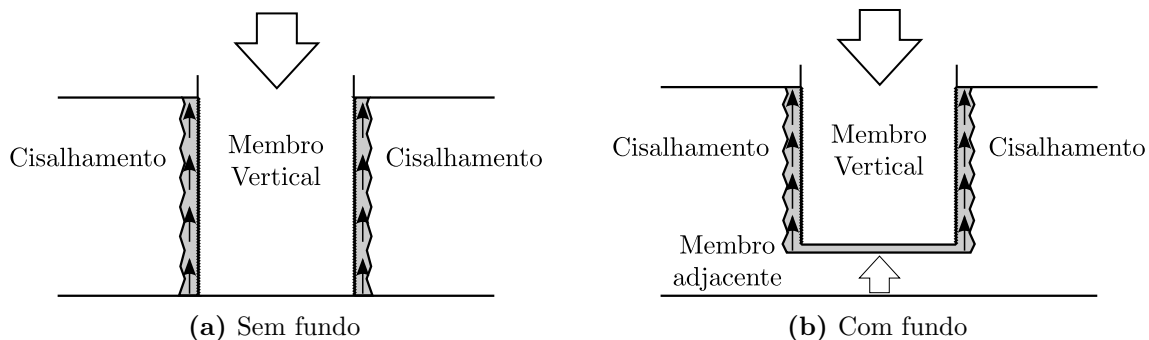
Figura 2.29 – Força axial em cálice embutido
