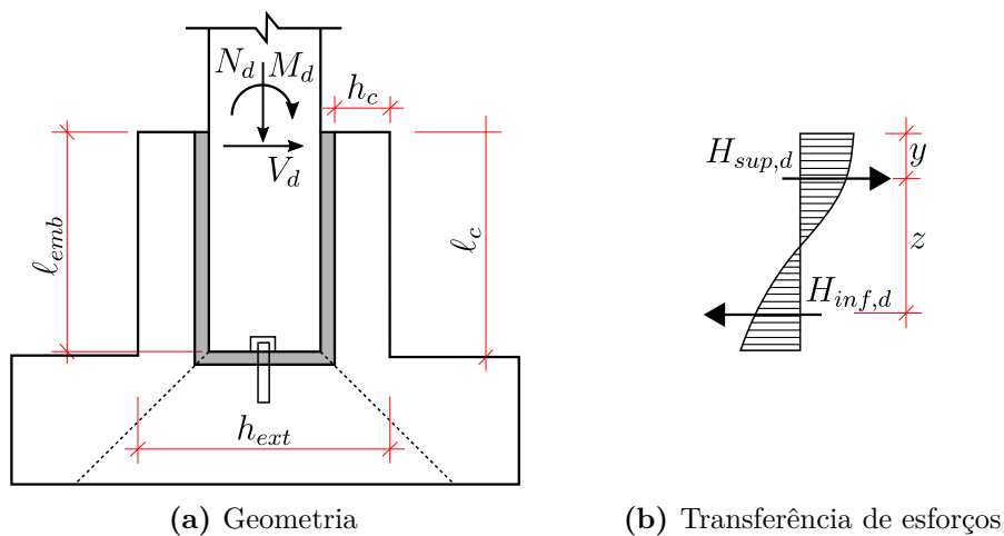
Figura 2.13 – Modelo de cálice liso de Leonhardt e Mönnig (1978)
