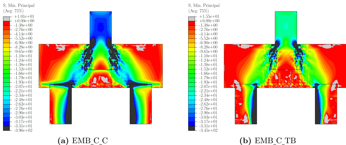
Figura 4.50 – Bielas de compressão dos blocos com cálice embutido de interface com chave de cisalhamento (MPa)
