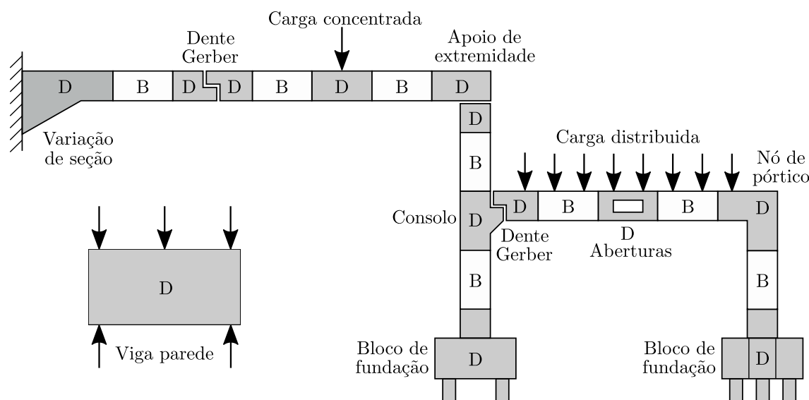
Figura 2.2 – Exemplos de regiões B e D
