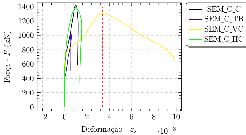
Figura 4.45 – Curvas força-deformação nas armaduras verticais dos cálices semiembutidos de interface com chave de cisalhamento
