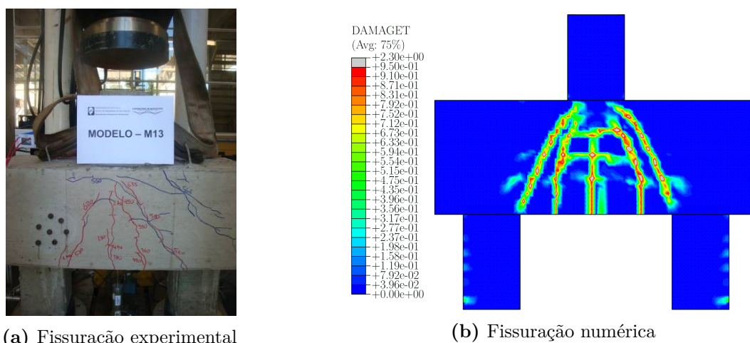
Figura 3.83 – Panorama de fissuração do modelo EMB_C
