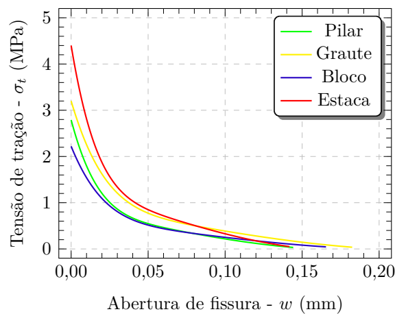
Figura 3.27 – Diagrama tensão-abertura de fissura nos concretos
