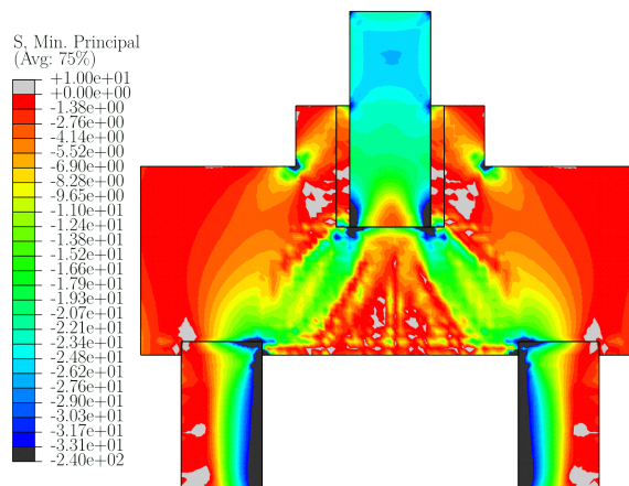
Figura 3.53 – Bielas de compressão do modelo SEM_AC_L (MPa)
