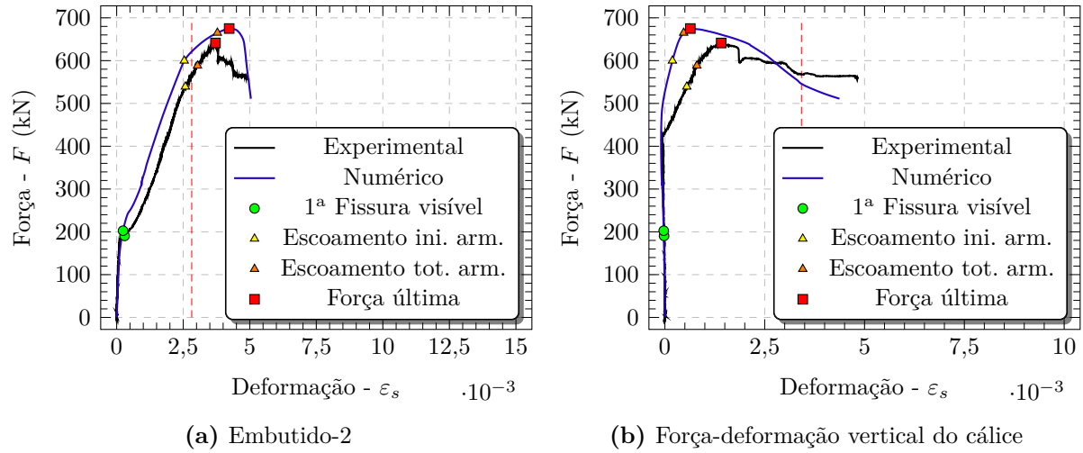
Figura 3.86 – Força-deformação das armaduras principais do modelo EMB_AC_C
