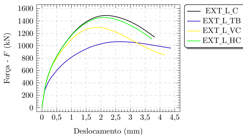
Figura 4.5 – Curvas força-deslocamento dos blocos com cálice externo de interface lisa
