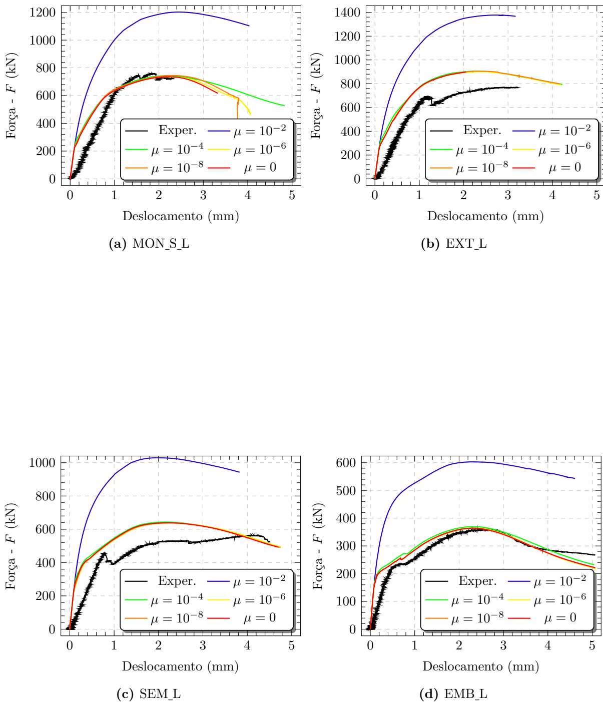
Figura 3.22 – Influência da viscosidade \mu na curva força-deslocamento dos modelos
