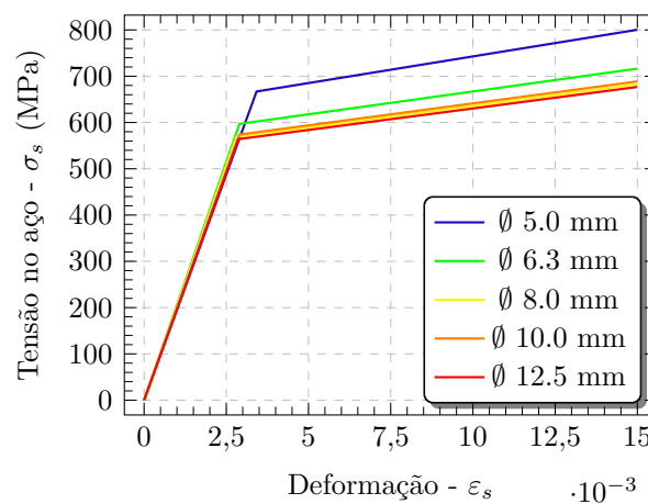
Figura 3.12 – Modelo tensão-deformação das barras de aço
