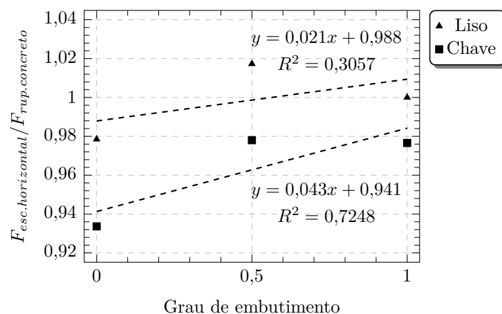
Figura 4.61 – Influência da armadura horizontal do cálice nos modelos
