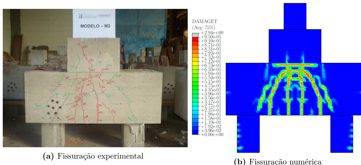
Figura 3.47 – Panorama de fissuração do modelo EXT_L
