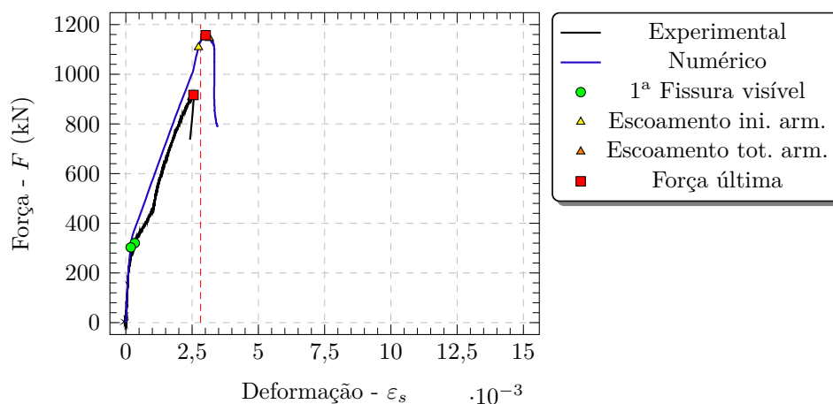
Figura 3.70 – Força-deformação tirante do bloco do modelo EXT_C
