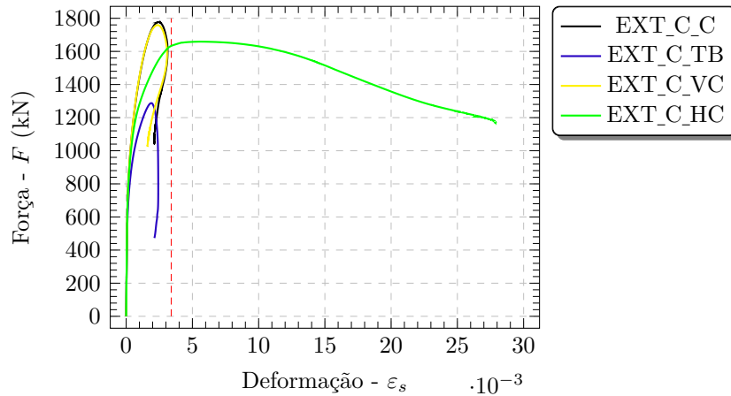
Figura 4.39 – Curvas força-deformação nas armaduras horizontais dos cálices externos de interface com chave de cisalhamento
