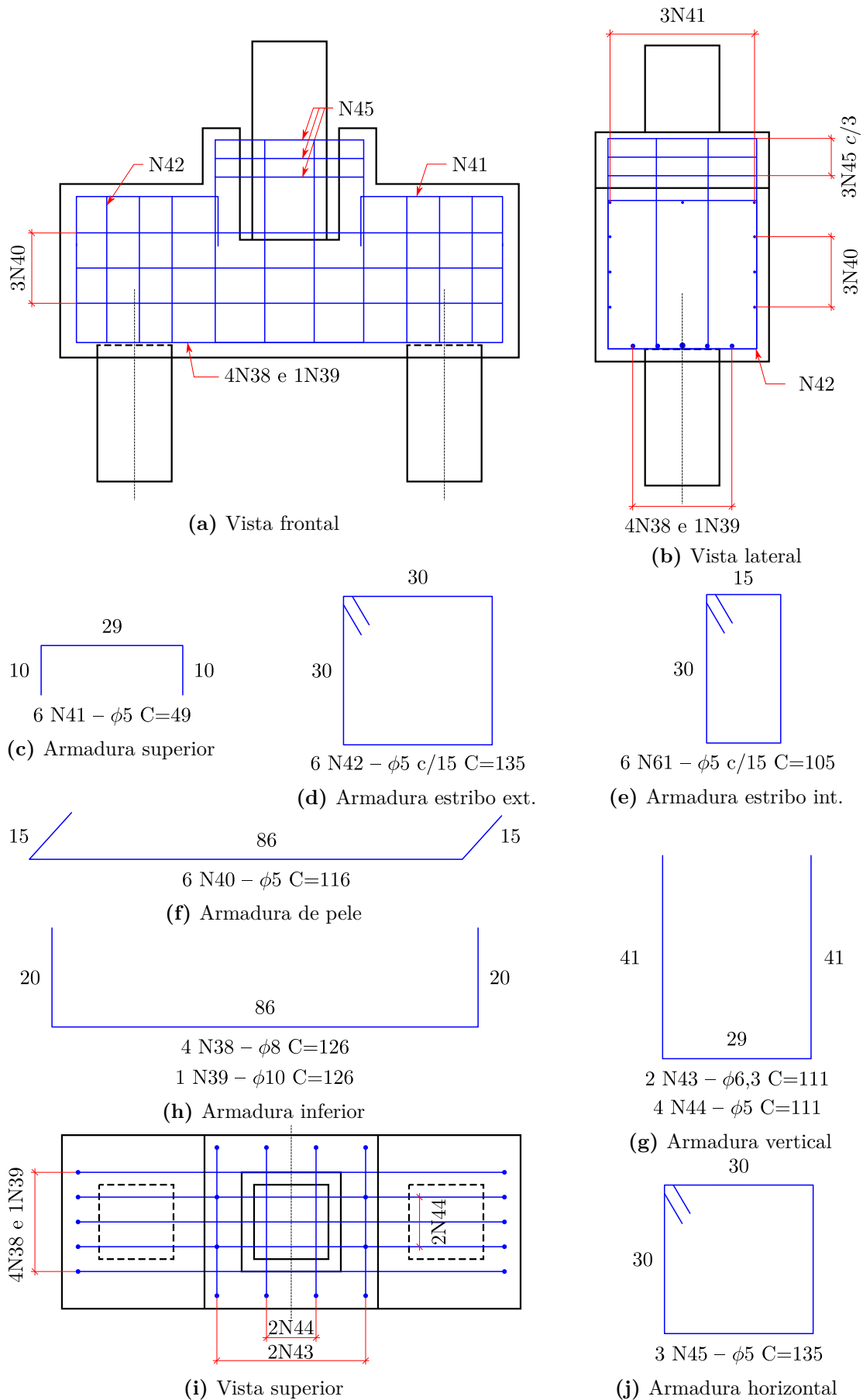
Figura A.9 – Detalhamento do bloco semiembutido liso (cm)
