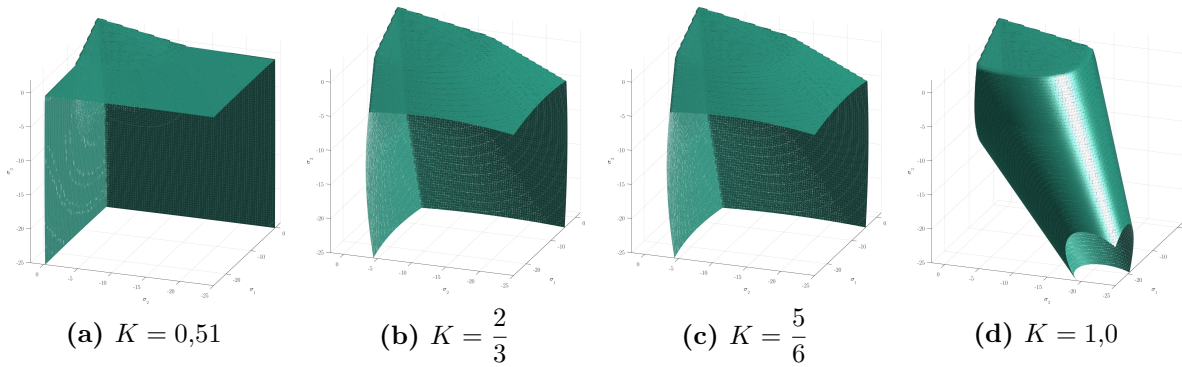
Figura 3.15 – Influência do parâmetro K na superfície de plastificação do CDP no espaço tridimensional de tensões principais
