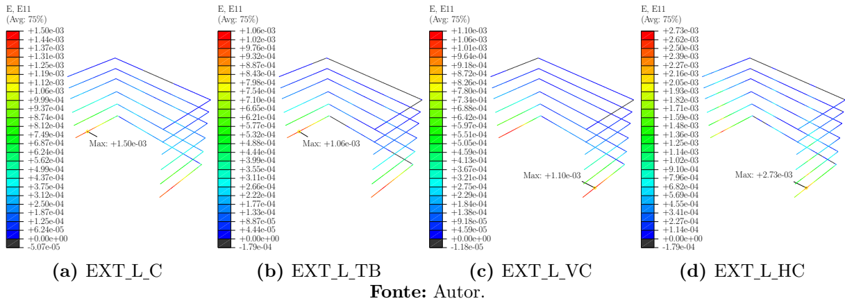
Figura 4.12 – Distribuição de deformações nas armaduras horizontais dos cálices externos de interface lisa
