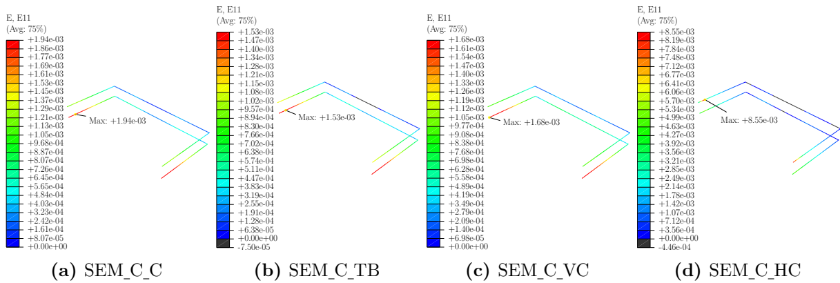
Figura 4.48 – Distribuição de deformações nas armaduras horizontais dos cálices semiembutidos de interface com chave de cisalhamento
