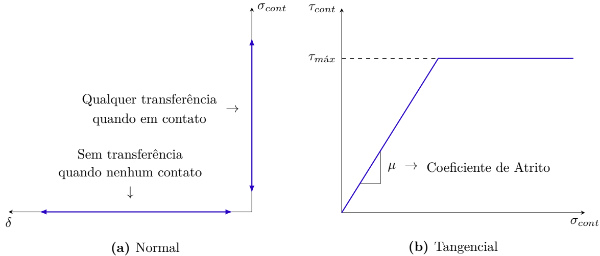
Figura 3.30 – Comportamento do contato
