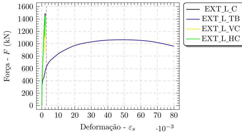
Figura 4.7 – Curvas força-deformação nos tirantes principais dos blocos com cálice externo de interface lisa
