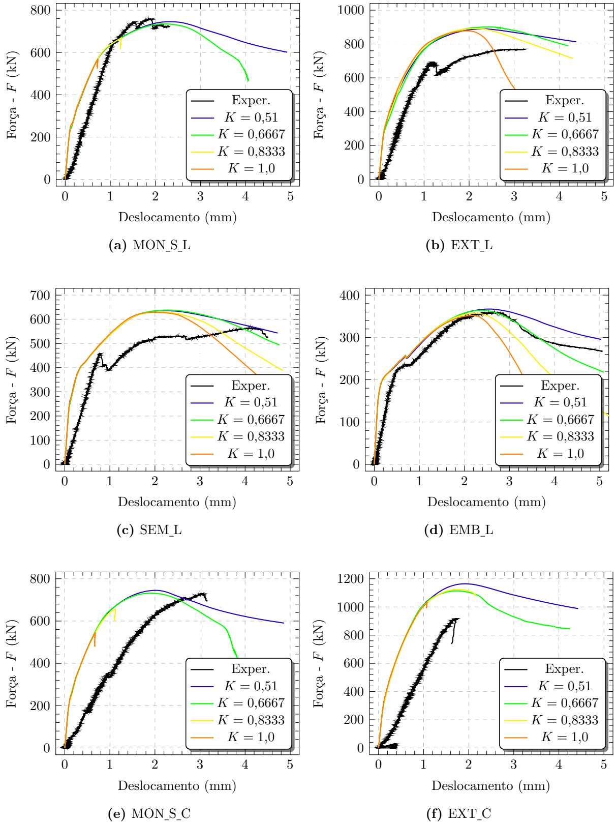
Figura 3.16 – Influência do parâmetro K na curva força-deslocamento dos modelos
