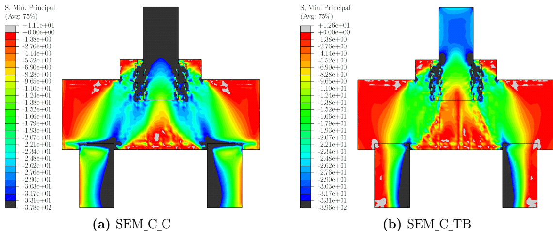
Figura 4.42 – Bielas de compressão dos blocos com cálice semiembutido de interface com chave de cisalhamento (MPa)
