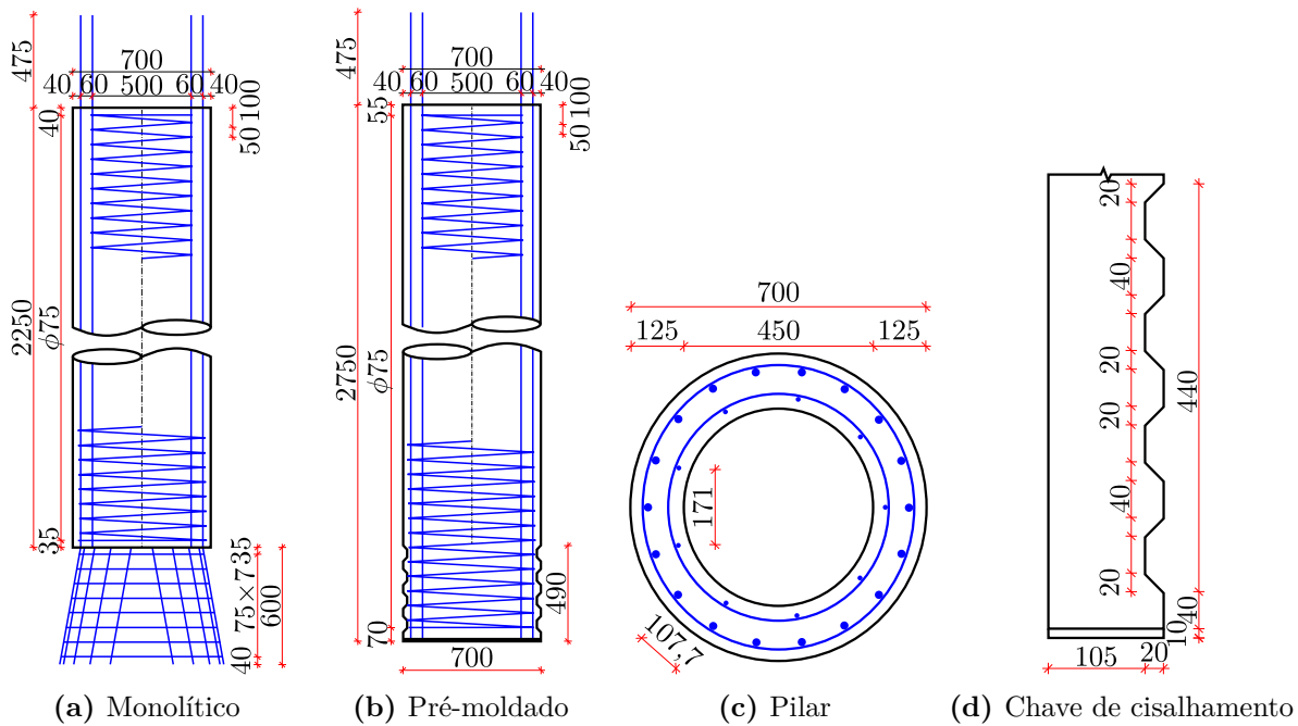
Figura 2.18 – Detalhes dos modelos testados (un: mm)
