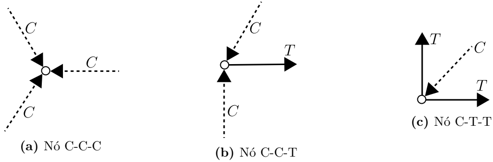
Figura 2.6 – Classificação dos nós
