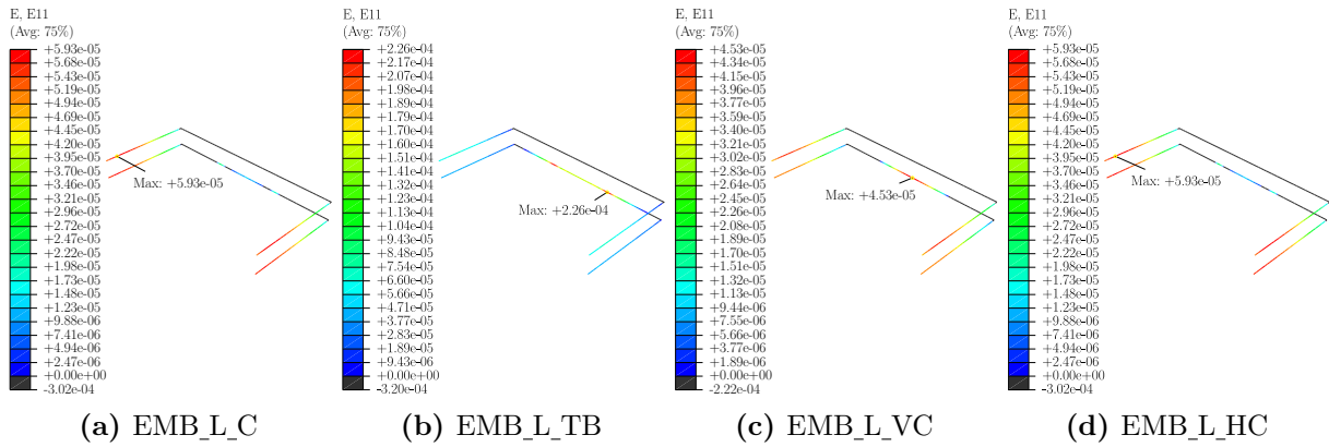
Figura 4.28 – Distribuição de deformações nas armaduras horizontais dos cálices embutidos de interface lisa
