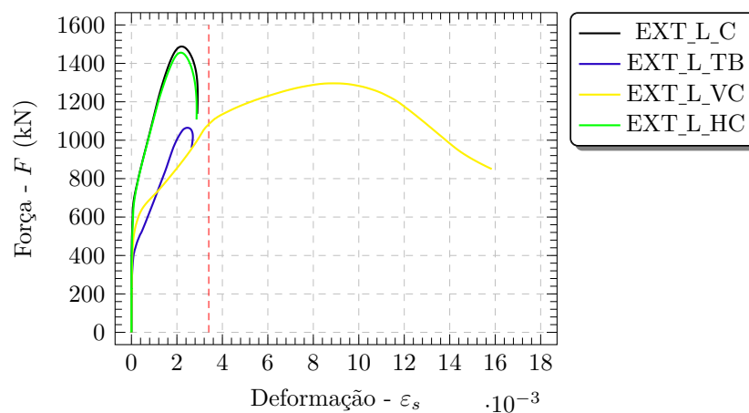
Figura 4.9 – Curvas força-deformação nas armaduras verticais dos cálices externos de interface lisa
