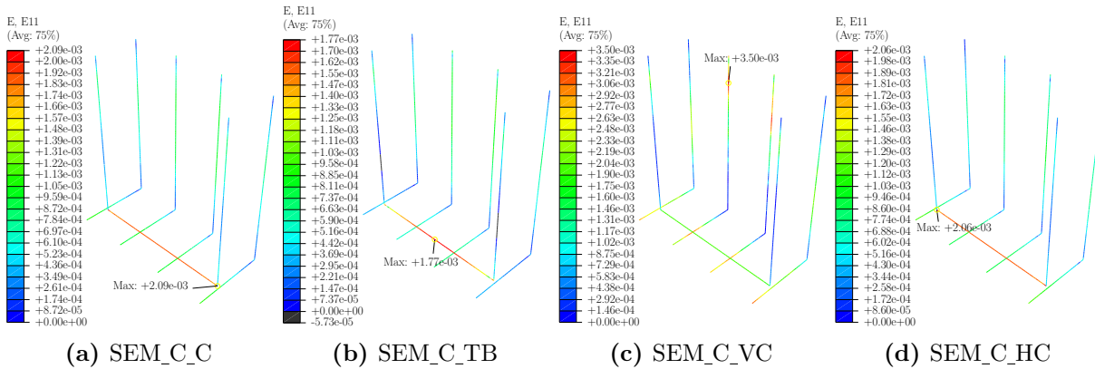
Figura 4.46 – Distribuição de deformações nas armaduras verticais dos cálices semiembutidos de interface com chave de cisalhamento
