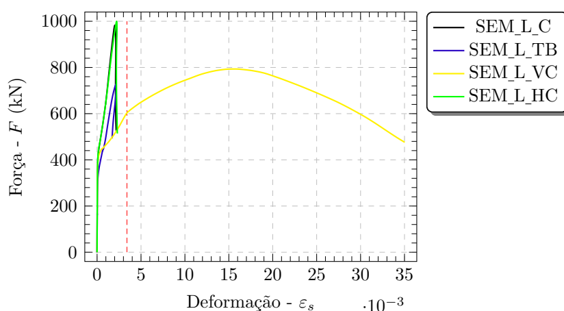
Figura 4.17 – Curvas força-deformação nas armaduras verticais dos cálices semiembutidos de interface lisa
