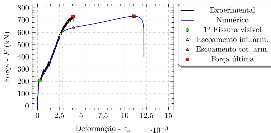
Figura 3.66 – Força-deformação tirante do bloco do modelo MON_S_C
