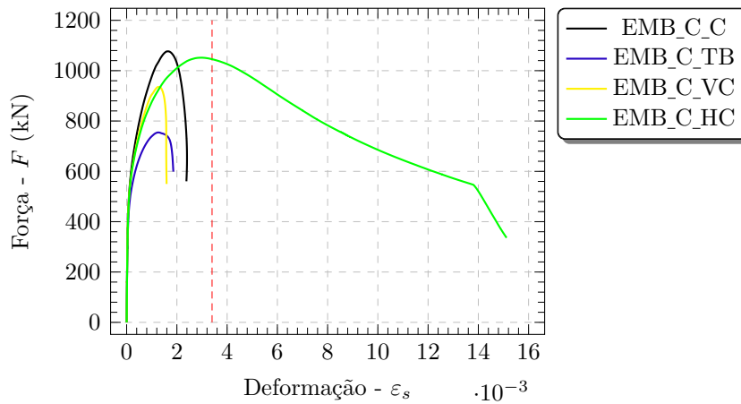
Figura 4.55 – Curvas força-deformação nas armaduras horizontais dos cálices embutidos de interface com chave de cisalhamento
