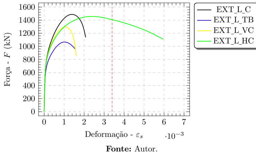
Figura 4.11 – Curvas força-deformação nas armaduras horizontais dos cálices externos de interface lisa
