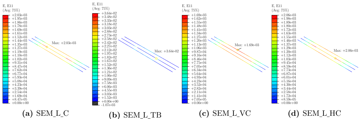
Figura 4.16 – Distribuição de deformação nos tirantes principais dos blocos com cálice semiembutido de interface lisa
