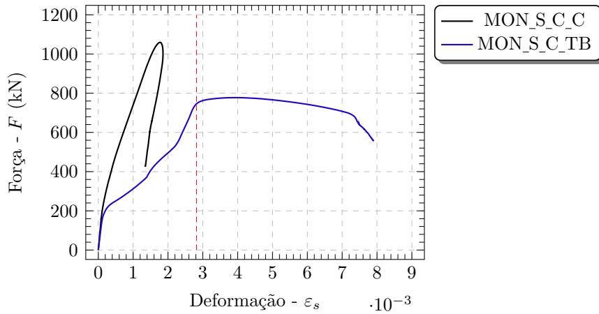
Figura 4.31 – Curvas força-deformação nos tirantes principais dos blocos monolíticos de referência da série com chave de cisalhamento
