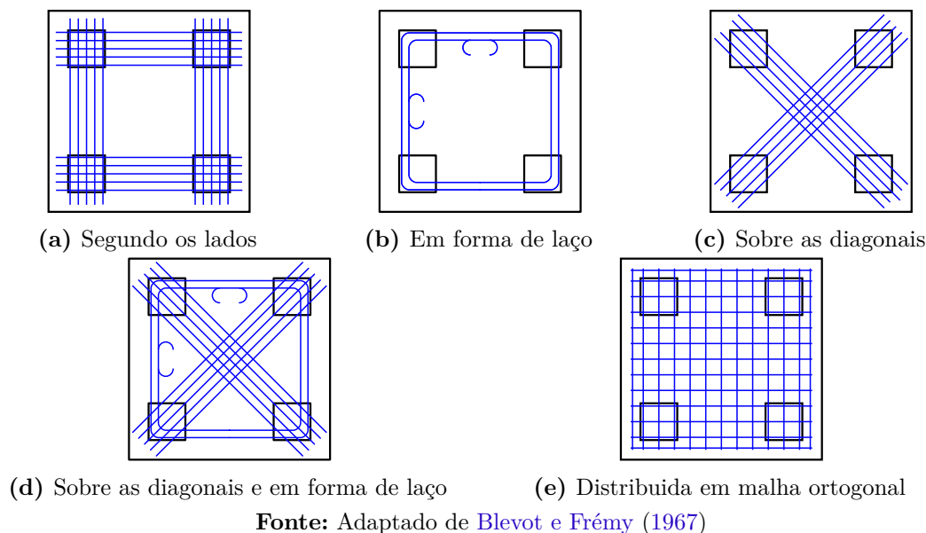
Figura 2.10 – Arranjo de armaduras em blocos de quatro estacas de Blevot e Frémy (1967)
