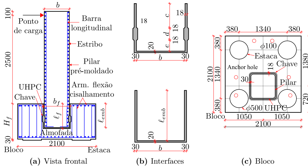
Figura 2.22 – Dimensões e detalhes estruturais dos modelos (un: mm)
