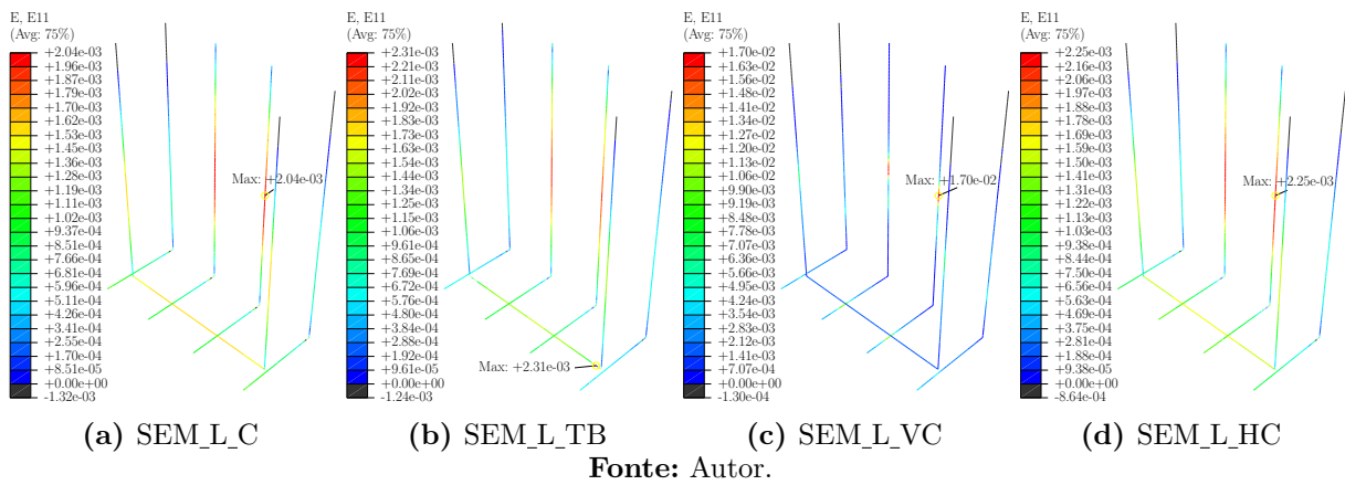
Figura 4.18 – Distribuição de deformações nas armaduras verticais dos cálices semiembutidos de interface lisa
