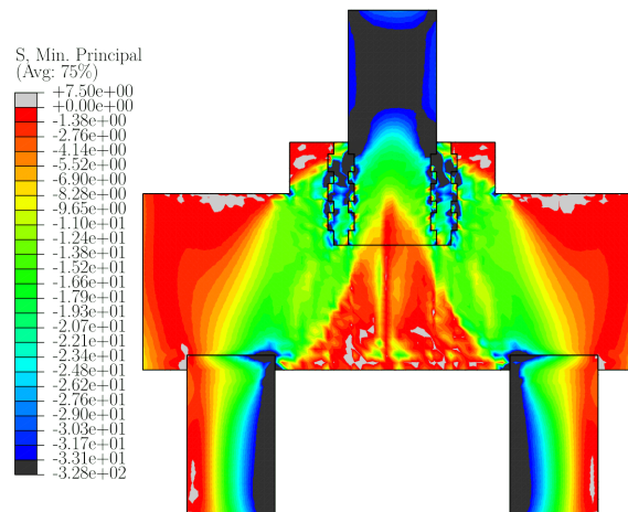
Figura 3.77 – Bielas de compressão do modelo SEM_AC_C (MPa)
