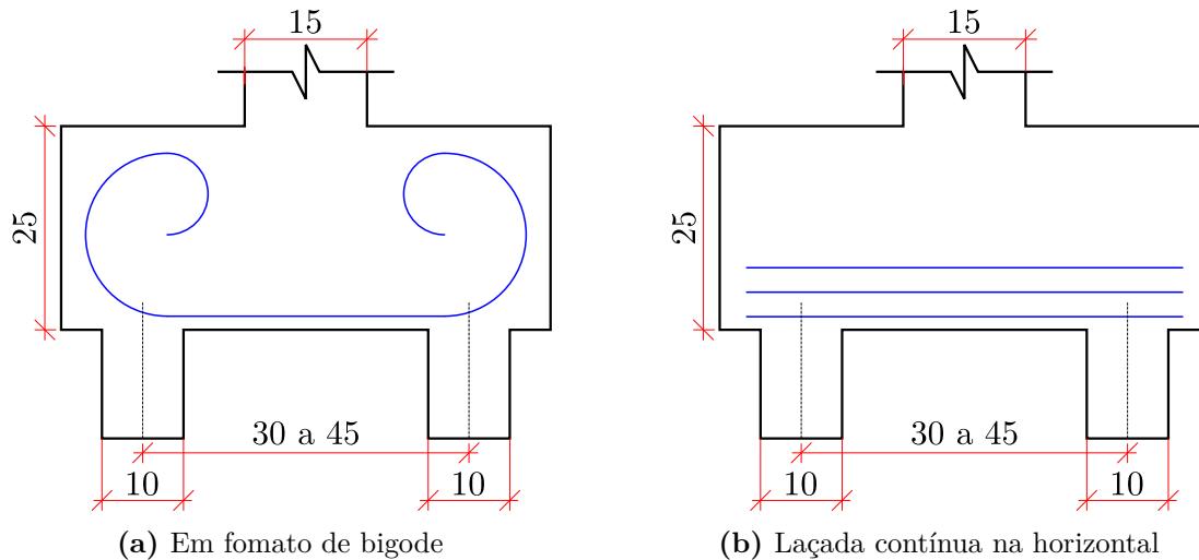
Figura 2.11 – Modelos de blocos sobre duas estacas ensaiados por Mautoni (1972)
