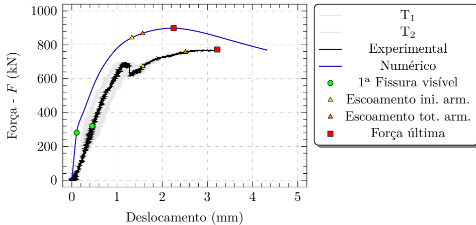
Figura 3.44 – Força-deslocamento do modelo EXT_L
