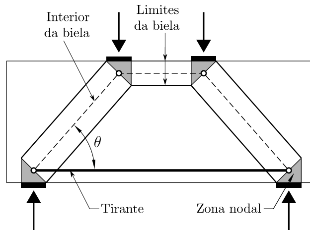
Figura 2.4 – Modelo de biela e tirante
