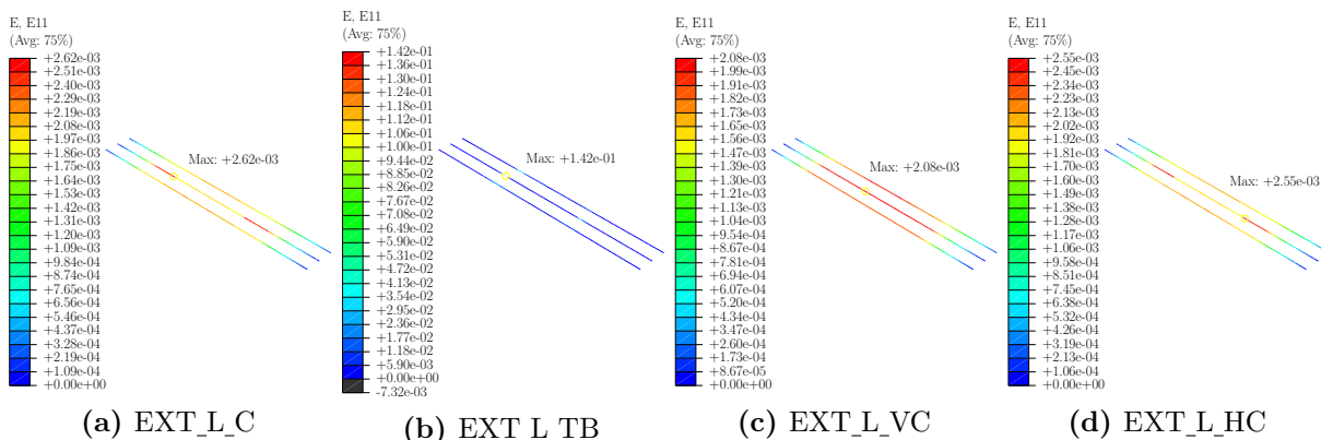
Figura 4.8 – Distribuição de deformação nos tirantes principais dos blocos com cálice externo de interface lisa
