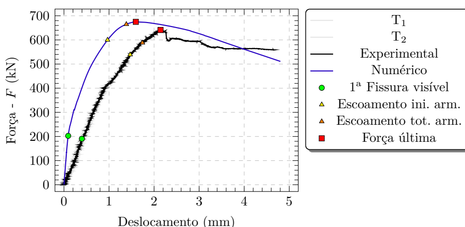
Figura 3.84 – Força-deslocamento do modelo EMB_AC_C
