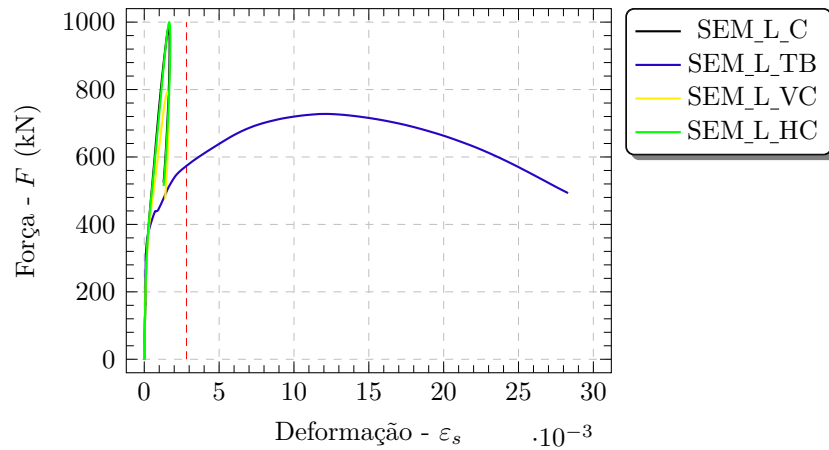
Figura 4.15 – Curvas força-deformação nos tirantes principais dos blocos com cálice semiembutido de interface lisa
