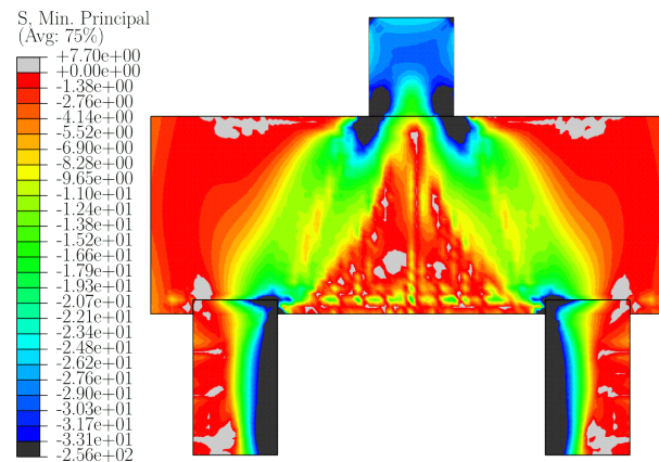
Figura 3.41 – Bielas de compressão do modelo MON_S_L (MPa)
