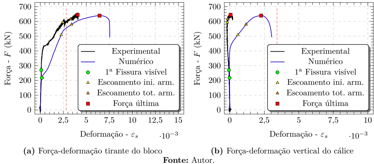
Figura 3.54 – Força-deformação nas armaduras principais do modelo SEM_AC_L
