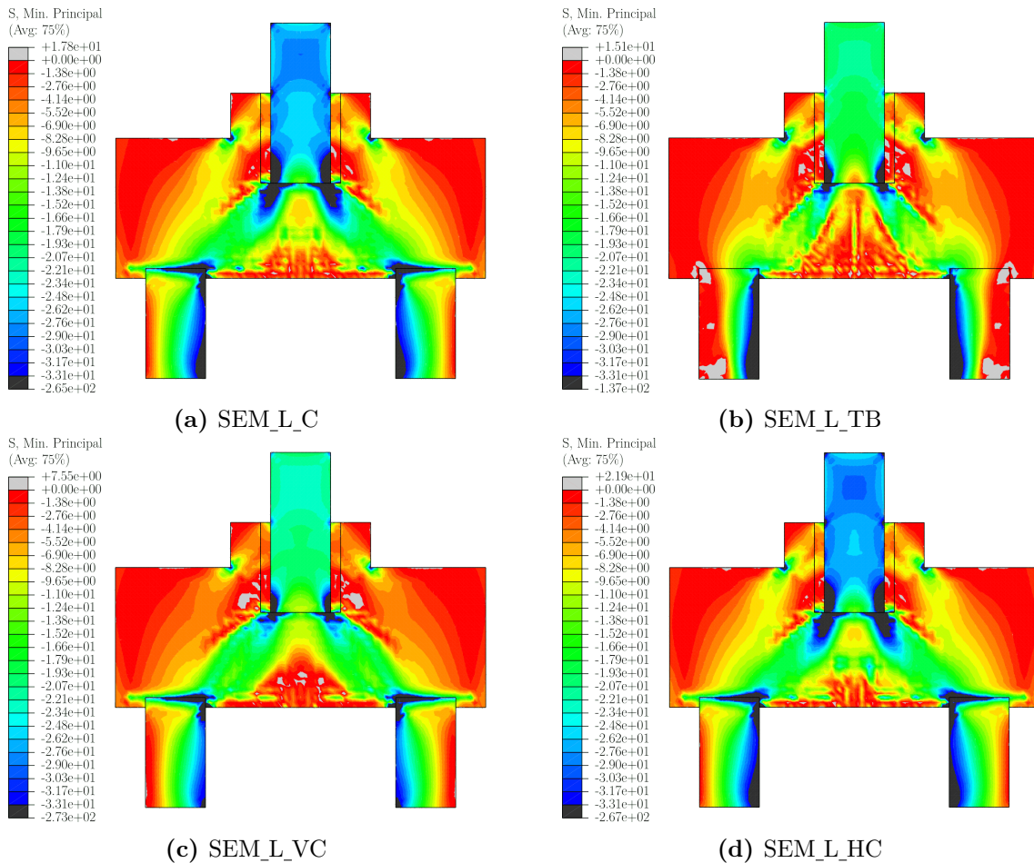
Figura 4.14 – Bielas de compressão dos blocos com cálice semiembutido de interface lisa (MPa)
