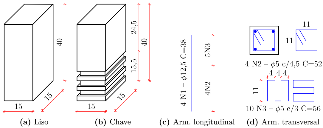
Figura A.2 – Propriedades geométricas dos pilares de concreto pré-moldado (cm)
