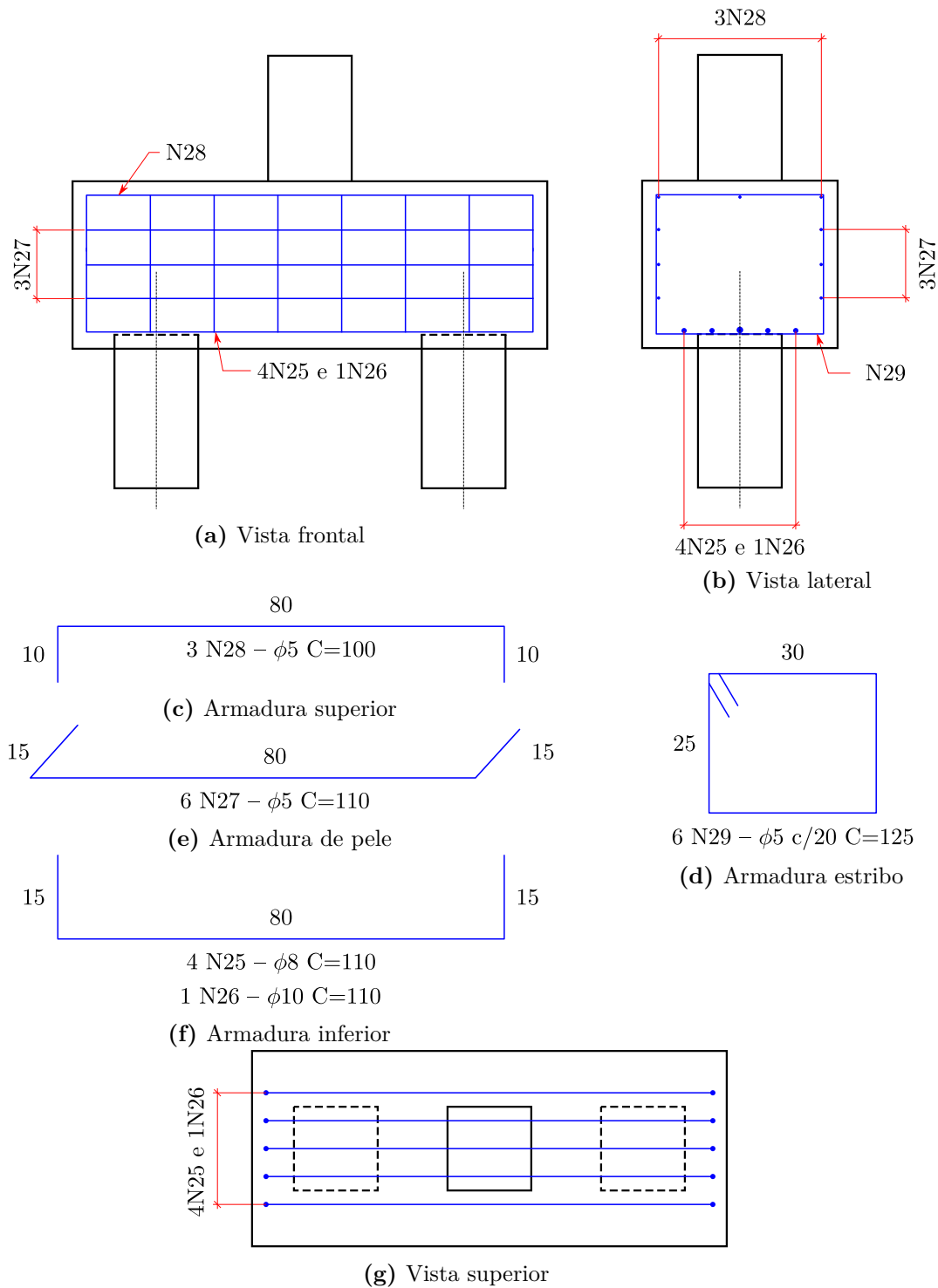
Figura A.13 – Detalhamento do bloco monolítico da série com chave de cisalhamento (cm)
