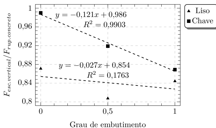
Figura 4.60 – Influência da armadura vertical do cálice nos modelos
