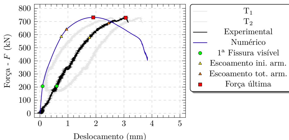
Figura 3.64 – Força-deslocamento do modelo MON_S_C
