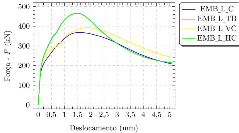
Figura 4.21 – Curvas força-deslocamento dos blocos com cálice embutido de interface lisa
