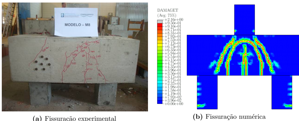
Figura 3.67 – Panorama de fissuração do modelo MON_S_C
