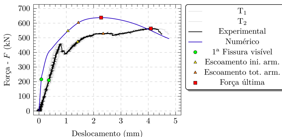
Figura 3.48 – Força-deslocamento do modelo SEM_L
