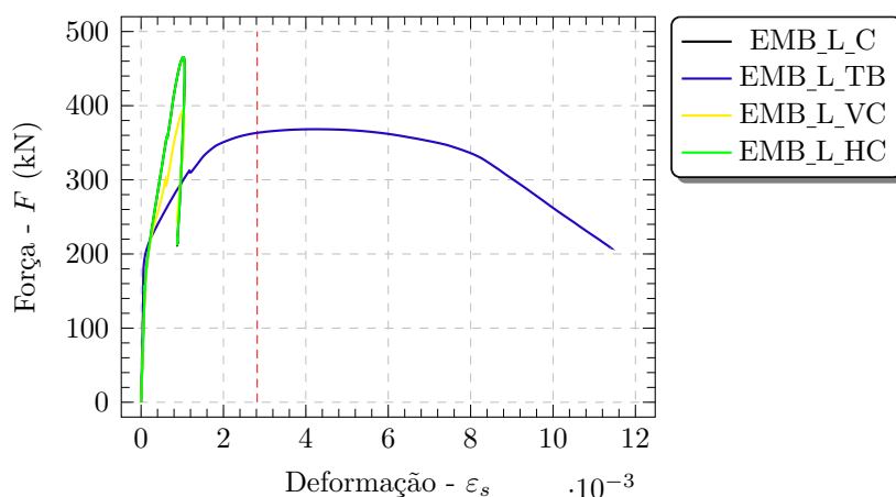
Figura 4.23 – Curvas força-deformação nos tirantes principais dos blocos com cálice embutido de interface lisa
