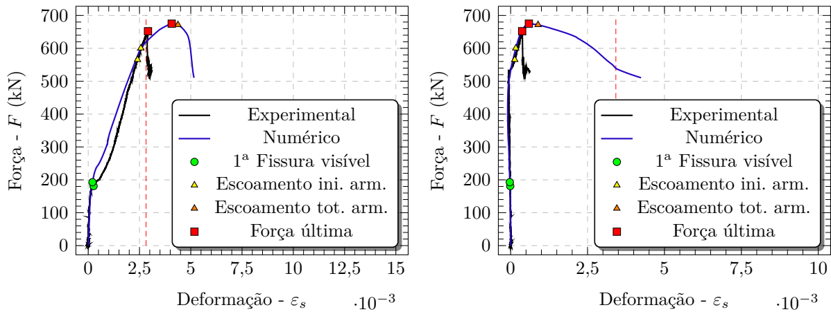
(a) Força-deformação tirante do bloco
