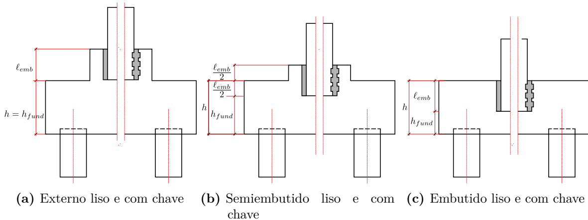
Figura 2.35 – Modelos ensaiados por Barros (2013)
