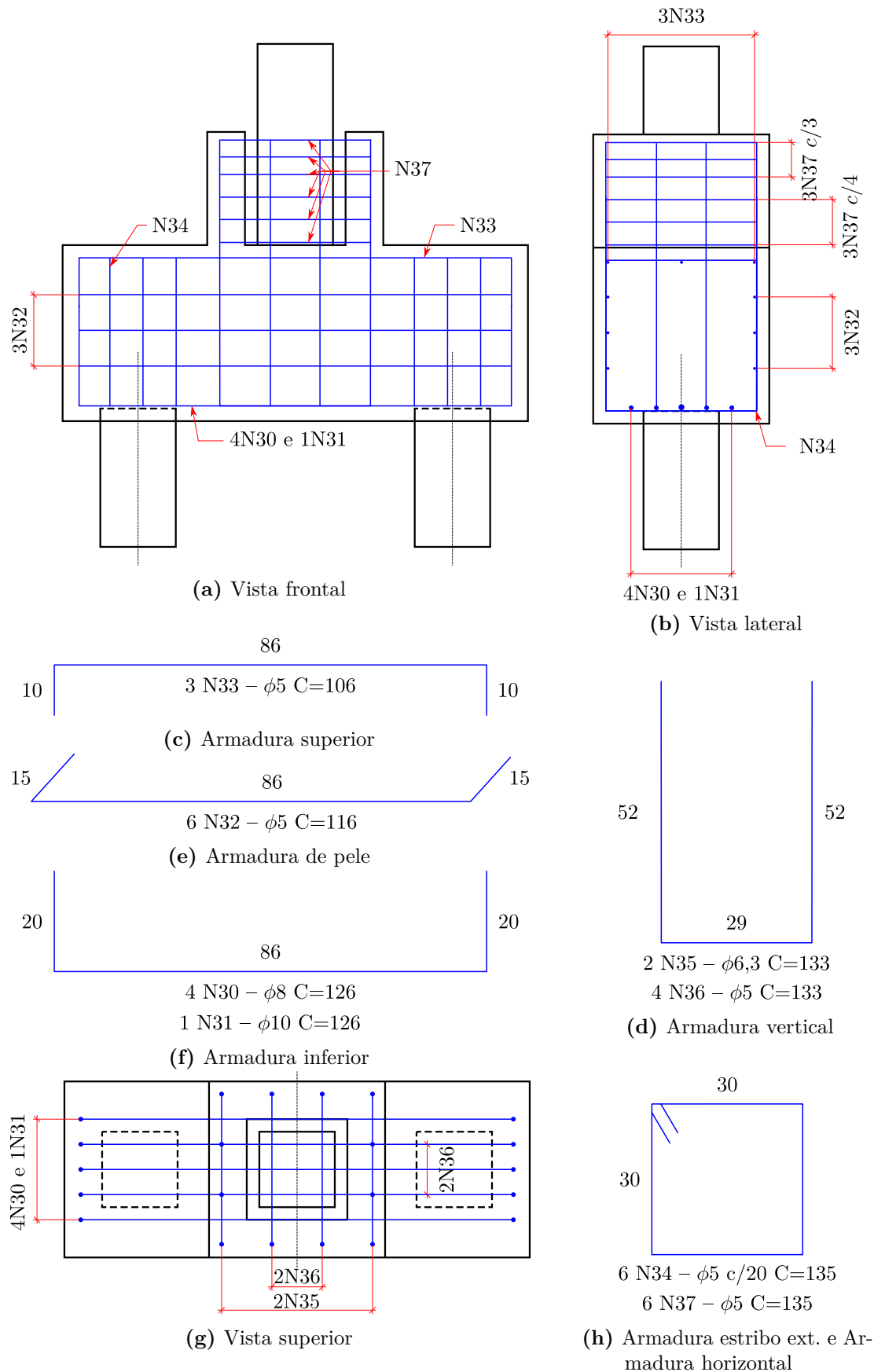
Figura A.7 – Detalhamento do bloco externo liso (cm)
