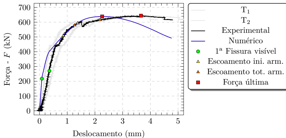
Figura 3.52 – Força-deslocamento do modelo SEM_AC_L
