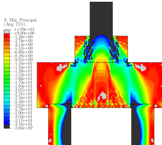
Figura 3.69 – Bielas de compressão do modelo EXT_C (MPa)
