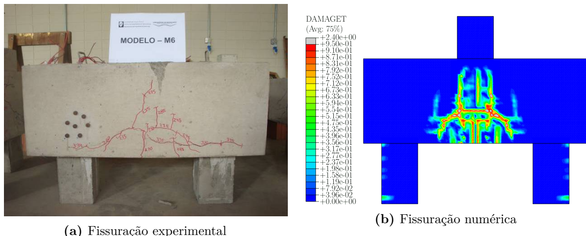
Figura 3.59 – Panorama de fissuração do modelo EMB_L
