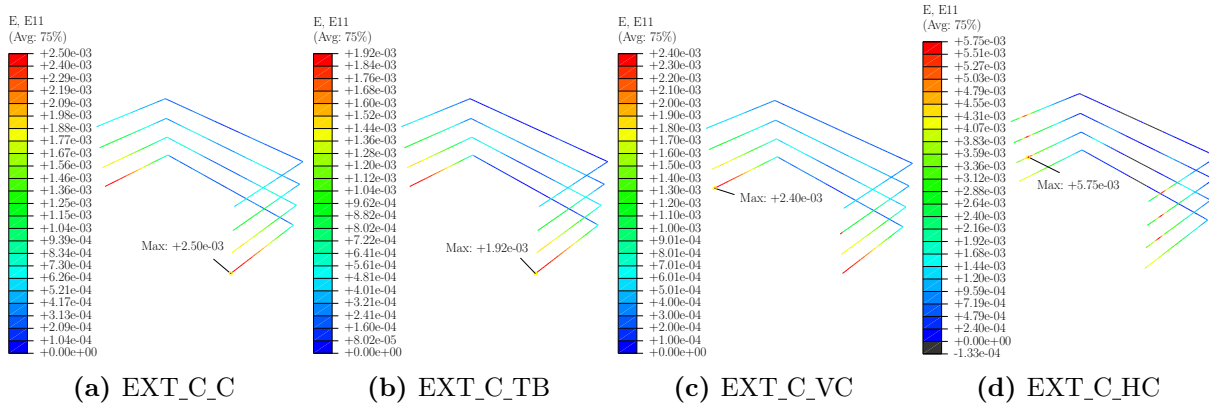
Figura 4.40 – Distribuição de deformações nas armaduras horizontais dos cálices externos de interface com chave de cisalhamento
