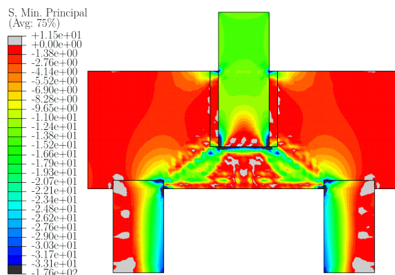
Figura 3.61 – Bielas de compressão do modelo EMB_AC_L (MPa)
