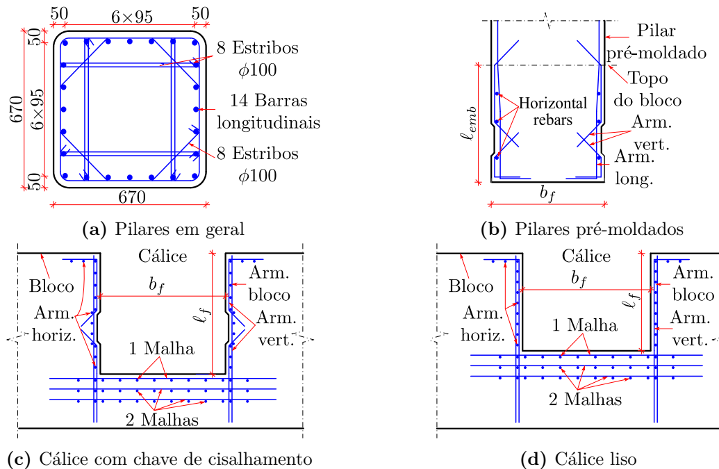
Figura 2.23 – Detalhamento (un: mm)
