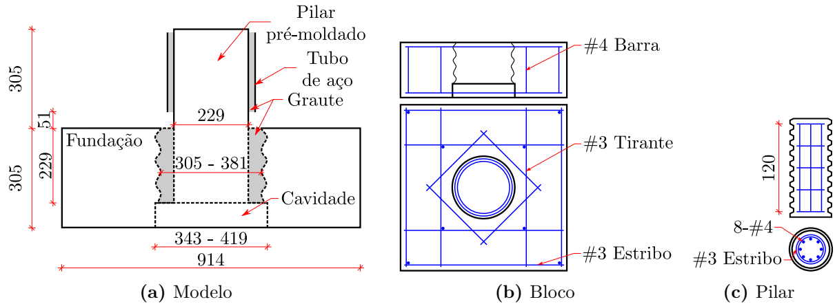
Figura 2.30 – Detalhes geométricos e das armações
