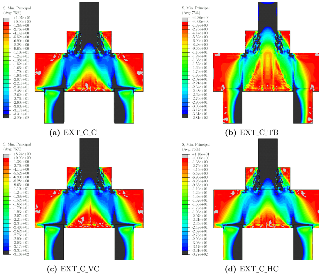
Figura 4.34 – Bielas de compressão dos blocos com cálice externo de interface com chave de cisalhamento (MPa)
