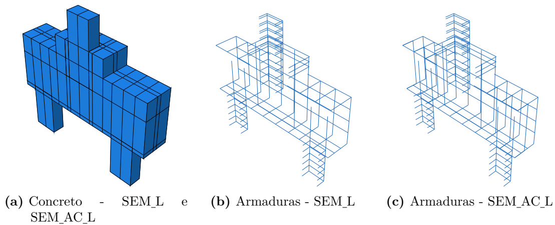
Figura 3.6 – Propriedades geométricas do bloco com cálice semiembutido da série lisa
