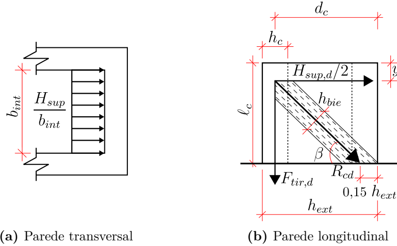
Figura 2.15 – Transferência de esforços segundo Leonhardt e Mönnig (1978)
