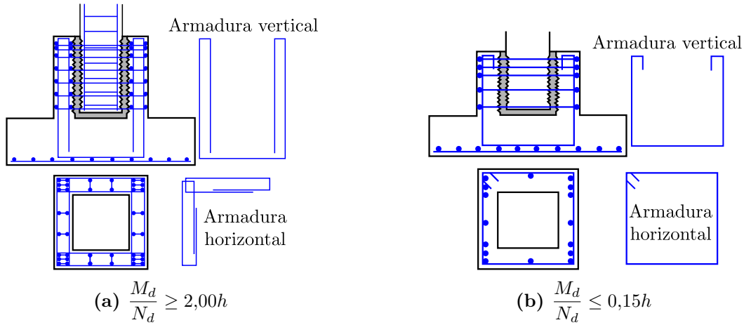
Figura 2.16 – Detalhamento das armaduras segundo Leonhardt e Mönnig (1978)
