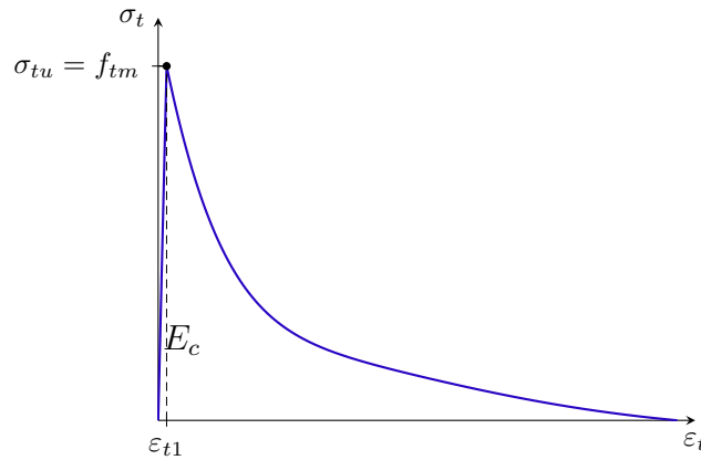
Figura 3.26 – Modelo do diagrama tensão-deformação à tração no concreto
