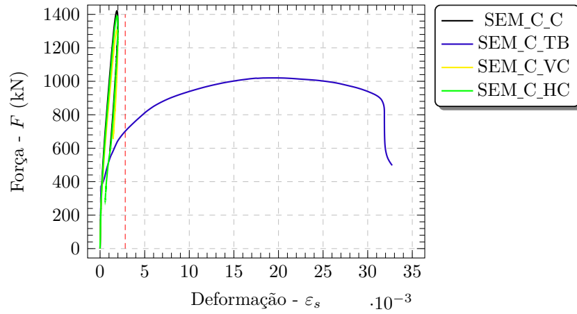
Figura 4.43 – Curvas força-deformação nos tirantes principais dos blocos com cálice semiembutidos de interface com chave de cisalhamento
