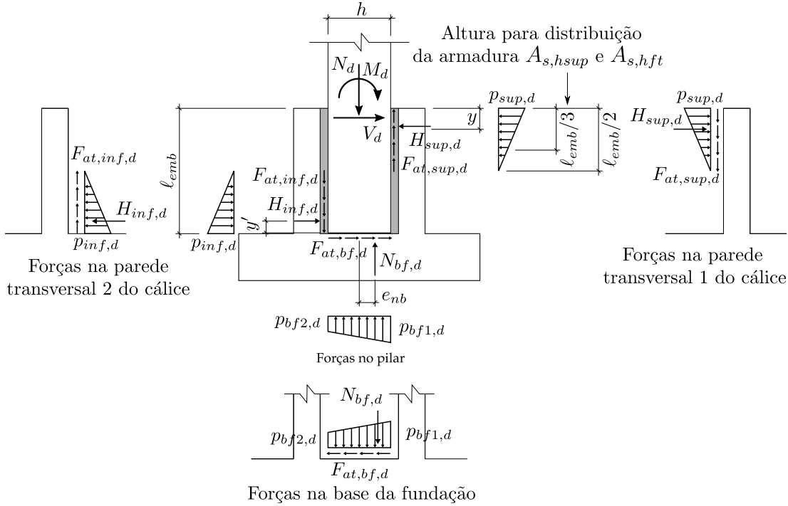
Figura 2.33 – Modelo de dimensionamento de cálice liso proposto por Canha (2004)
