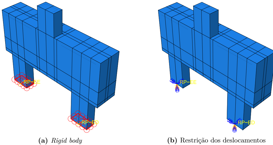
Figura 3.35 – Condição de contorno da base das estacas
