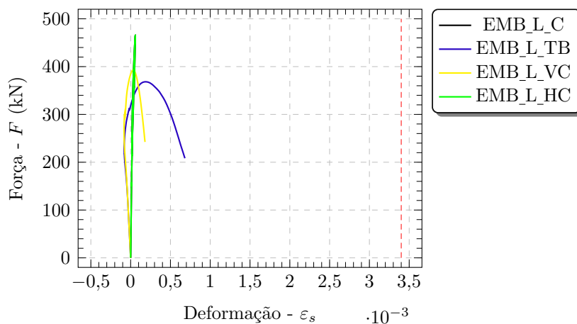
Figura 4.27 – Curvas força-deformação nas armaduras horizontal dos cálices embutidos lisos
