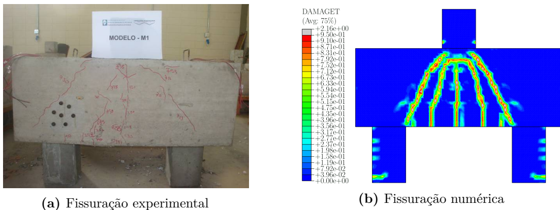
Figura 3.43 – Panorama de fissuração do modelo MON_S_L
