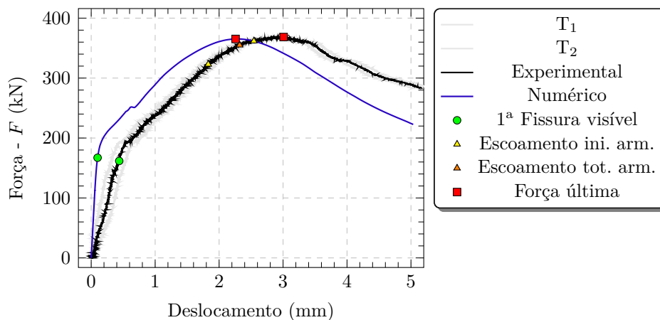
Figura 3.60 – Força-deslocamento do modelo EMB_AC_L
