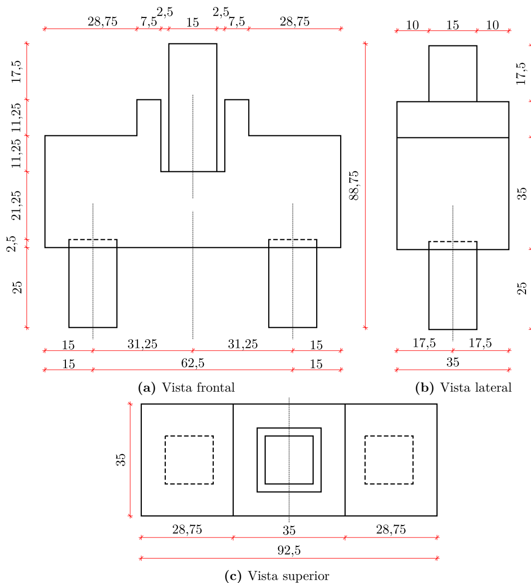
Figura A.8 – Propriedades geométricas do bloco com cálice semiembutido liso (cm)
