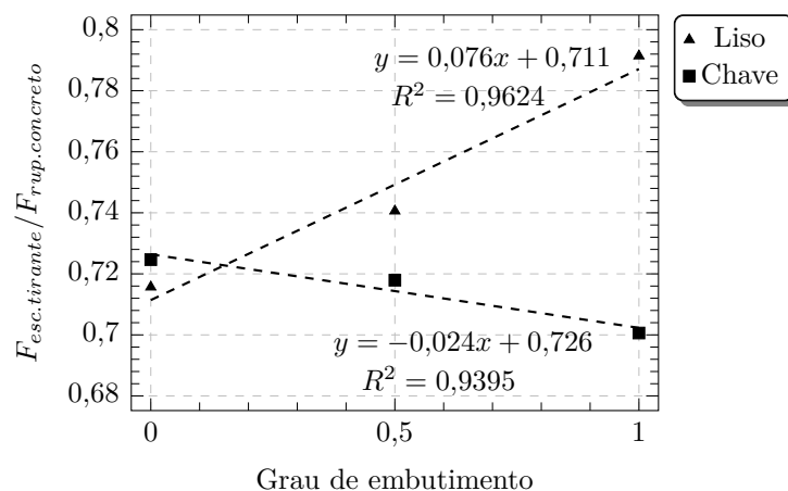
Figura 4.59 – Influência do tirante principal do bloco nos modelos
