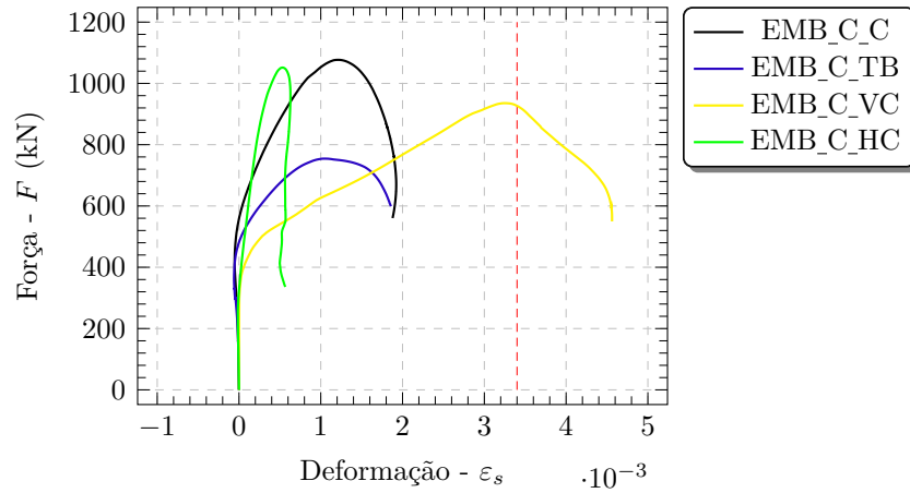
Figura 4.53 – Curvas força-deformação nas armaduras verticais dos cálices embutidos de interface com chave de cisalhamento
