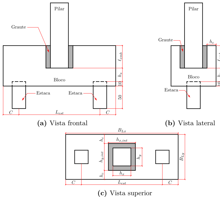
Figura 2.34 – Projeto do bloco sobre duas estacas ensaiados por Delalibera (2009)
