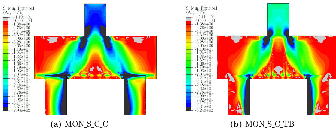
Figura 4.30 – Bielas de compressão dos blocos monolíticos de referência da série com chave de cisalhamento (MPa)
