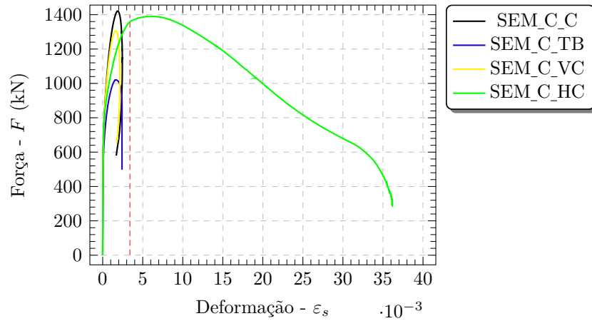
Figura 4.47 – Curvas força-deformação nas armaduras horizontais dos cálices semiembutidos de interface com chave de cisalhamento
