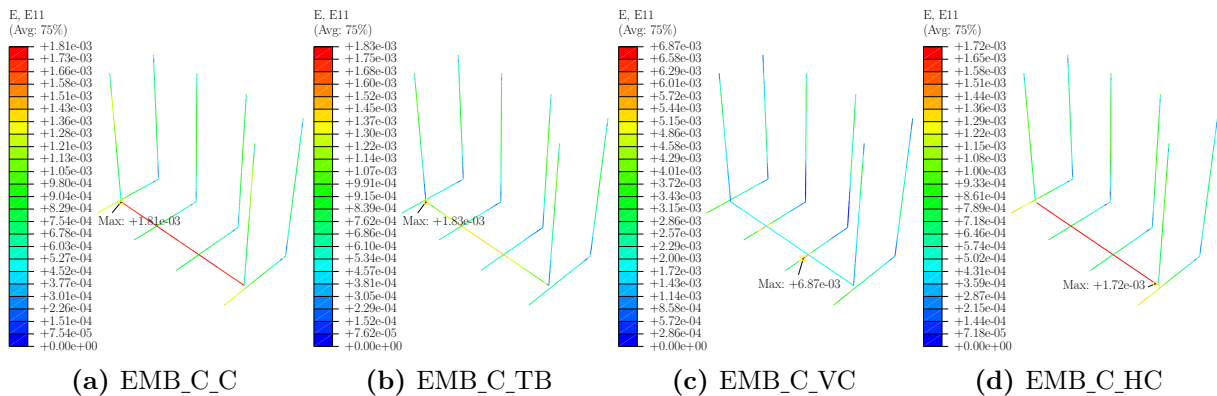
Figura 4.54 – Distribuição de deformações nas armaduras verticais dos cálices embutidos de interface com chave de cisalhamento
