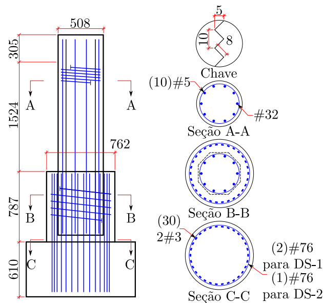
Figura 2.19 – Modelo simulado (un: cm)
