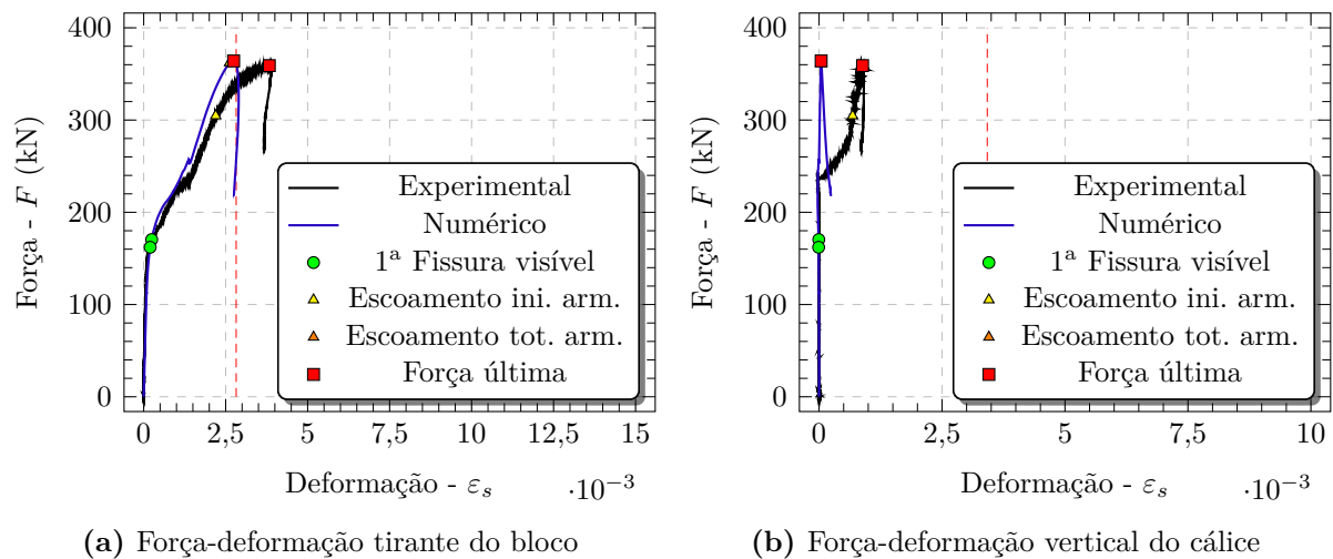
Figura 3.58 – Força-deformação nas armaduras principais do modelo EMB_L
