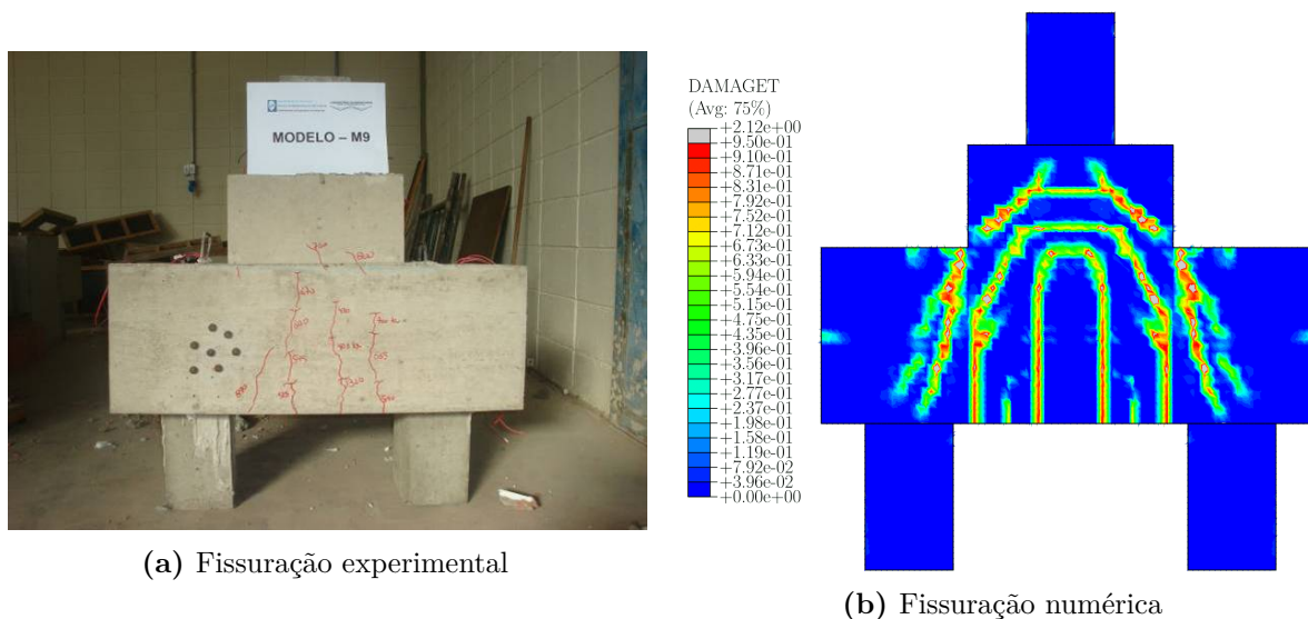
Figura 3.71 – Panorama de fissuração do modelo EXT_C
