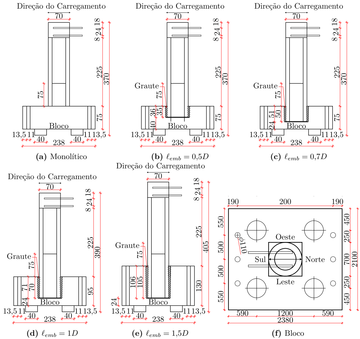
Figura 2.17 – Modelos testados (un: mm)
