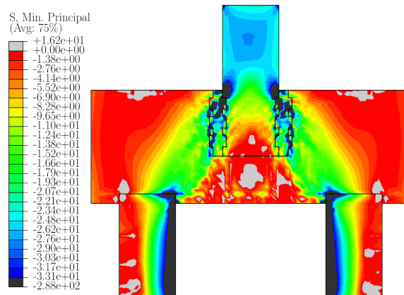
Figura 3.85 – Bielas de compressão do modelo EMB_AC_C (MPa)
