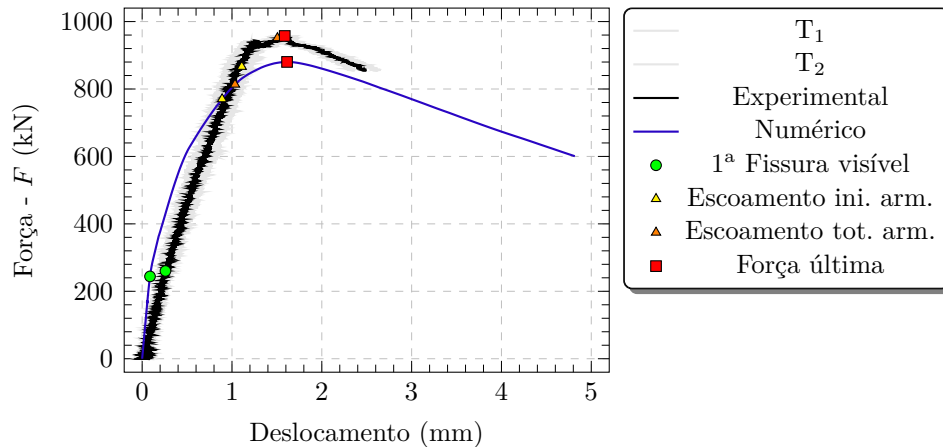
Figura 3.76 – Força-deslocamento do modelo SEM_AC_C
