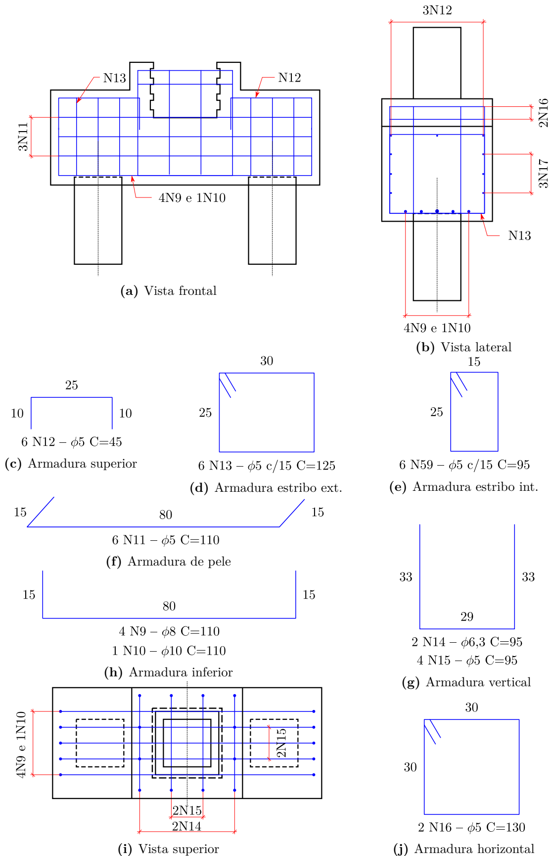
Figura A.17 – Detalhamento do bloco semiembutido da série com chave de cisalhamento (cm)
