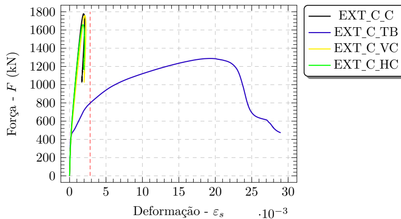
Figura 4.35 – Curvas força-deformação nos tirantes principais dos blocos com cálice externo de interface com chave de cisalhamento
