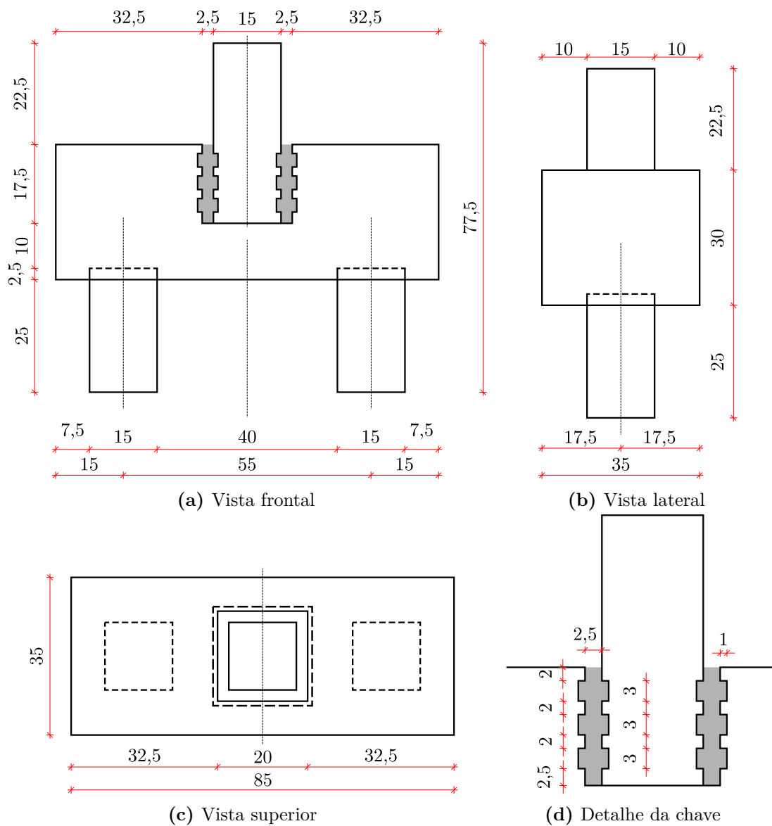
Figura A.18 – Propriedades geométricas do bloco com cálice embutido da série com chave de cisalhamento (cm)
