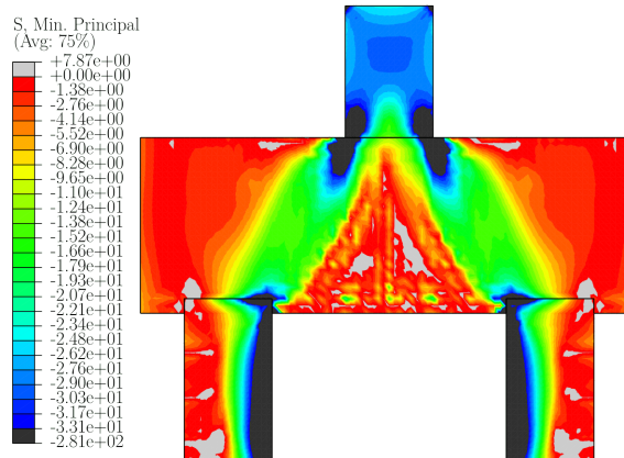
Figura 3.65 – Bielas de compressão do modelo MON_S_C (MPa)
