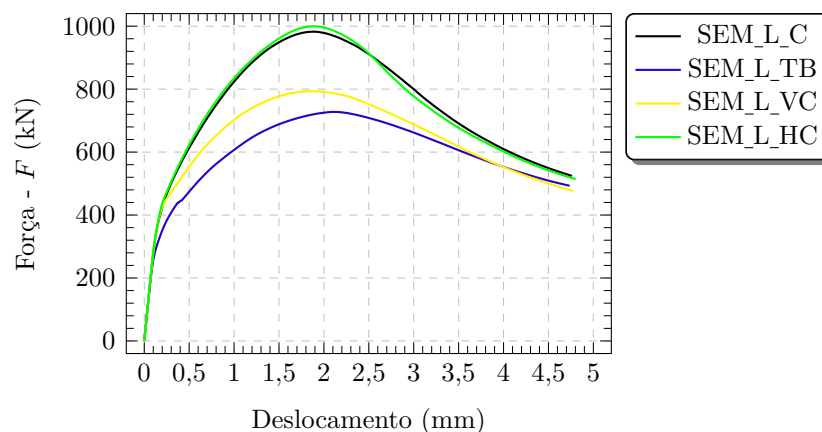
Figura 4.13 – Curvas força-deslocamento dos blocos com cálice semiembutido de interface lisa
