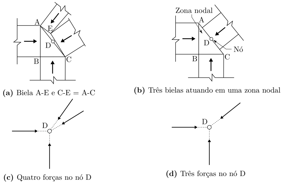
Figura 2.5 – Resultante das forças na zona nodal
