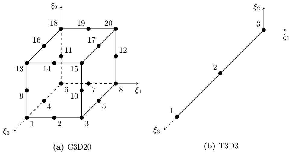
Figura 3.36 – Elementos finitos utilizados nos modelos numéricos
