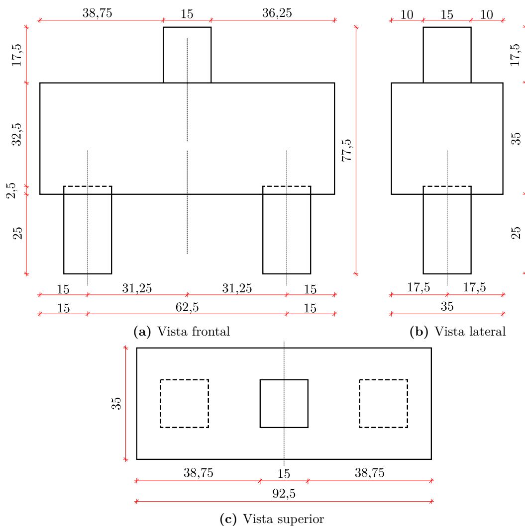
Figura A.4 – Propriedades geométricas do bloco monolítico da série lisa (cm)
