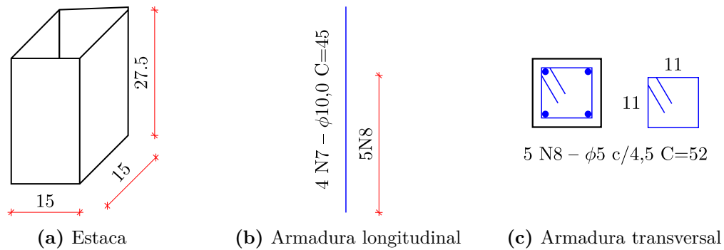
Figura A.3 – Propriedades geométricas das estacas (cm)
