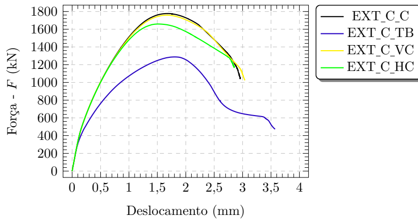
Figura 4.33 – Curvas força-deslocamento dos blocos com cálice externo de interface com chave de cisalhamento
