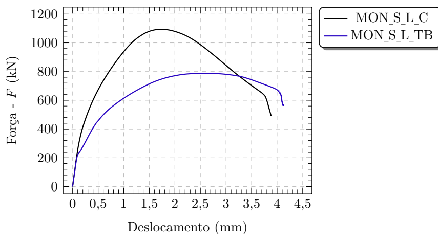
Figura 4.1 – Curvas força-deslocamento dos blocos monolíticos de referência da série lisa
