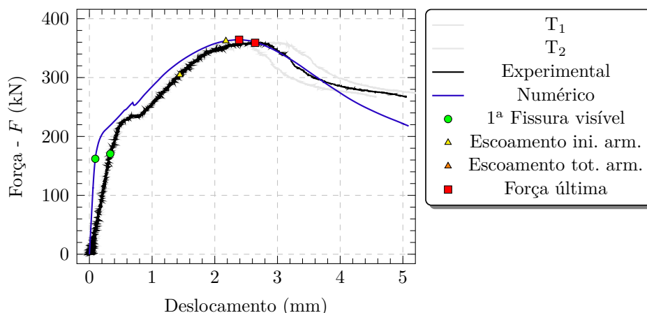
Figura 3.56 – Força-deslocamento do modelo EMB_L
