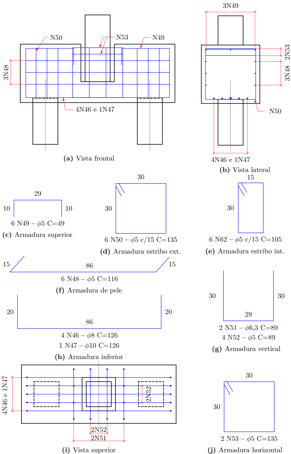
Figura A.11 – Detalhamento do bloco embutido liso (cm)
