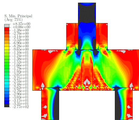
Figura 3.45 – Bielas de compressão do modelo EXT_L (MPa)
