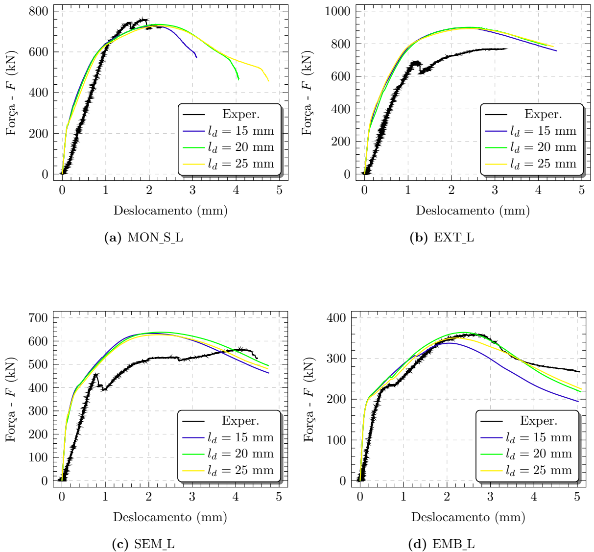
Figura 3.37 – Influência da malha no comportamento da curva força-deslocamento
