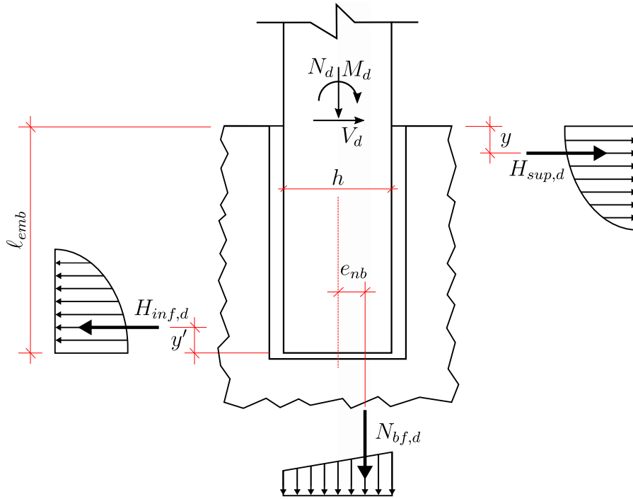
Figura 2.37 – Transferência dos esforços em cálices de interfaces lisas ou rugosas com grande excentricidade
