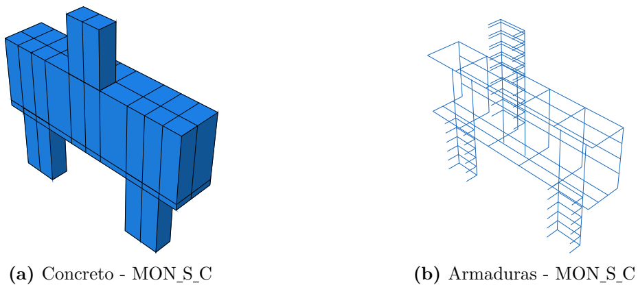
Figura 3.8 – Propriedades geométricas do bloco monolítico de referência da série com chave de cisalhamento
