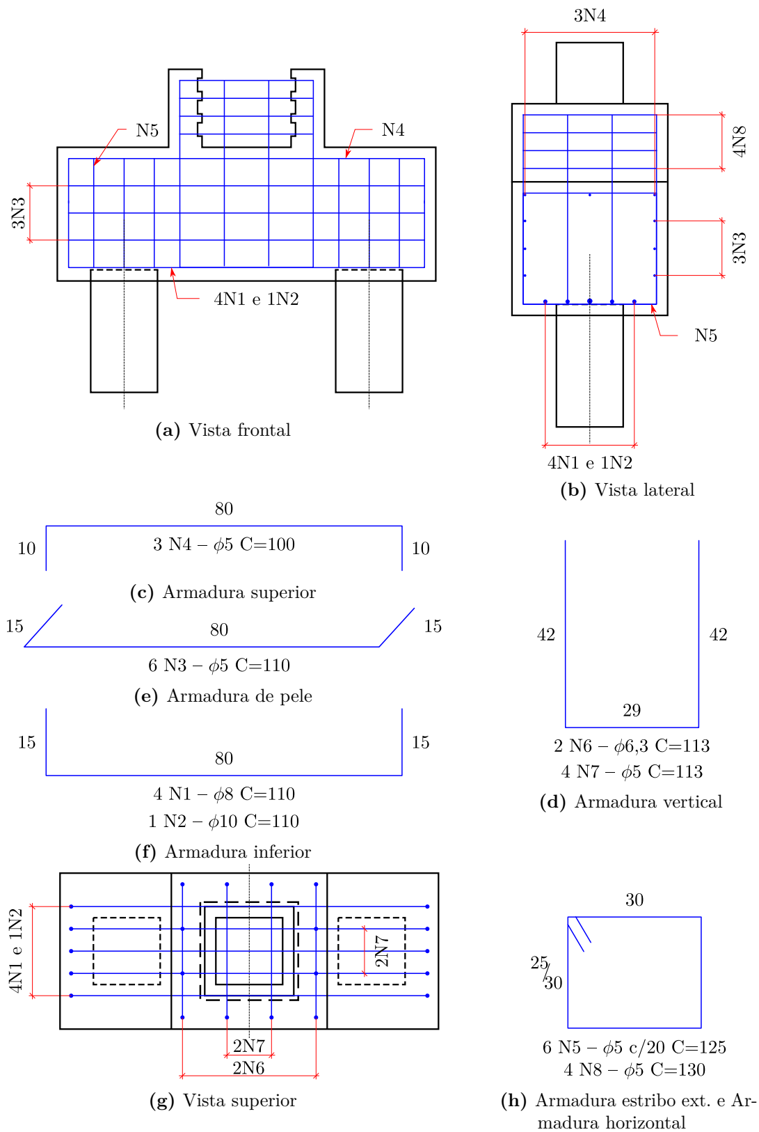
Figura A.15 – Detalhamento do bloco externo liso (cm)
