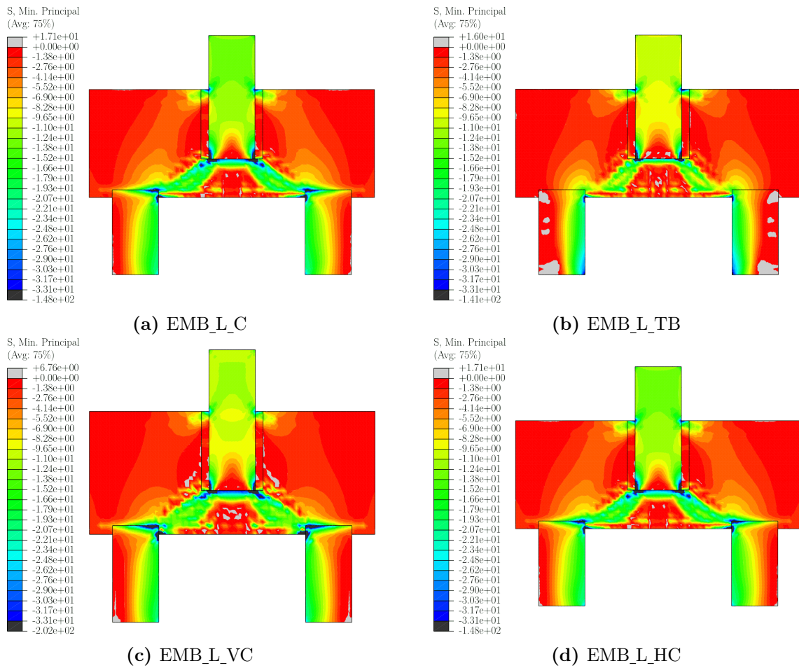
Figura 4.22 – Bielas de compressão dos blocos com cálice embutido de interface lisa (MPa)
