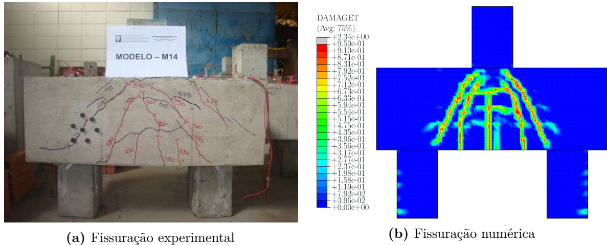
Figura 3.87 – Panorama de fissuração do modelo EMB_AC_C
