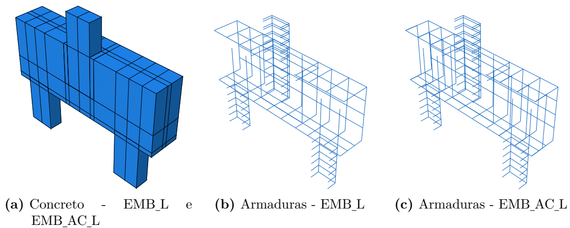
Figura 3.7 – Propriedades geométricas do bloco com cálice embutido da série lisa
