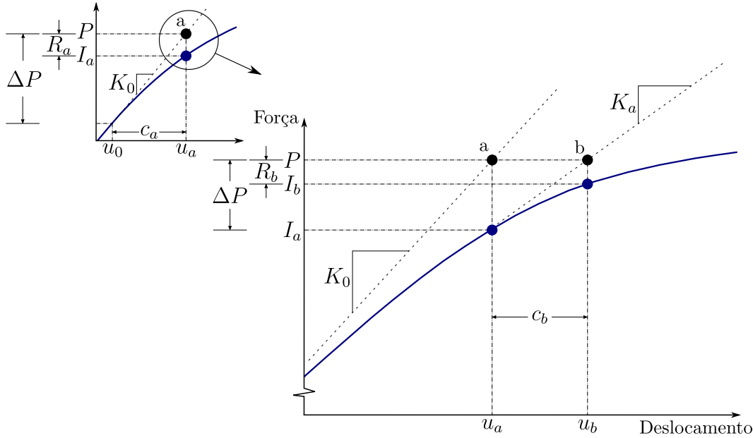
Figura 3.39 – Método iterativo e incremental de Newton-Raphson
