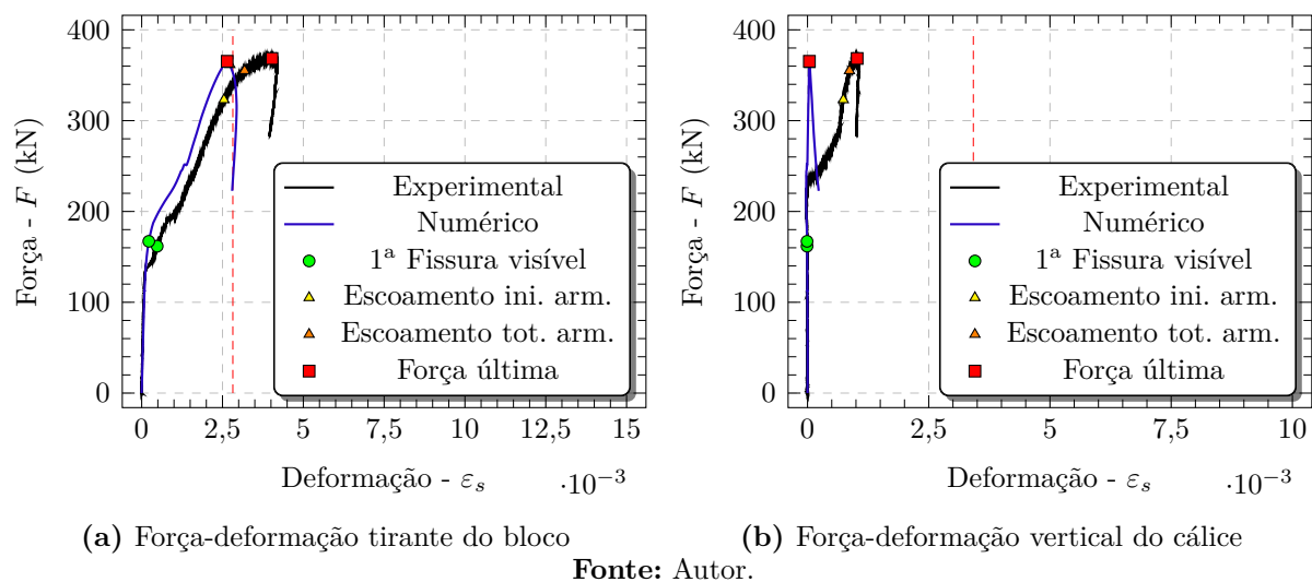
Figura 3.62 – Força-deformação nas armaduras principais do modelo EMB_AC_L
