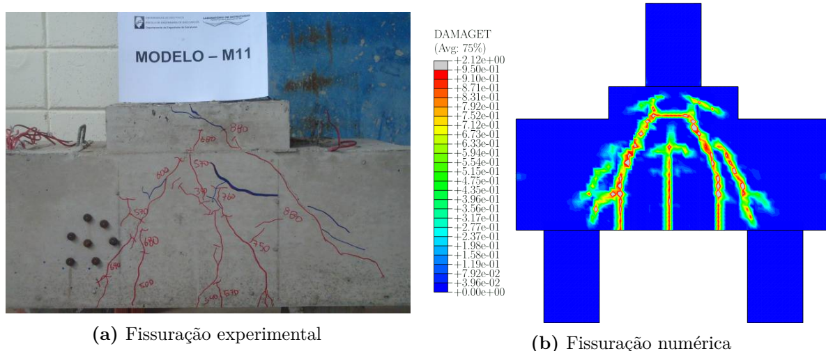
Figura 3.75 – Panorama de fissuração do modelo SEM_C
