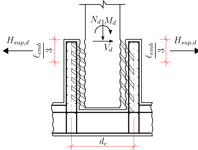
Figura 2.39 – Transferência dos esforços em cálices de interfaces com chaves de cisalhamento
