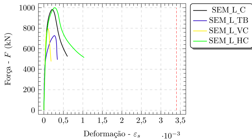
Figura 4.19 – Curvas força-deformação nas armaduras horizontais dos cálices semiembutidos de interface lisa
