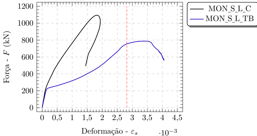
Figura 4.3 – Curvas força-deformação nos tirantes principais dos blocos monolíticos de referência da série lisa
