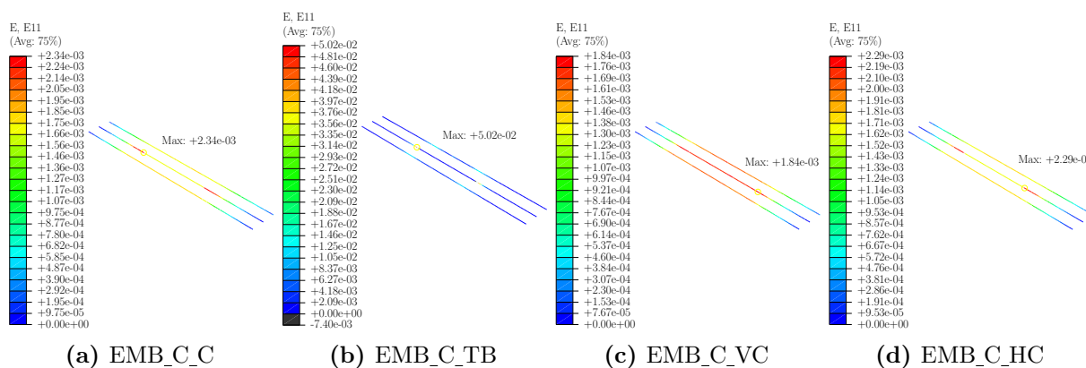
Figura 4.52 – Distribuição de deformações nos tirantes principais dos blocos com cálice embutido de interface com chave de cisalhamento
