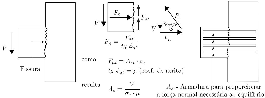
Figura 2.3 – Modelo de atrito-cisalhamento
