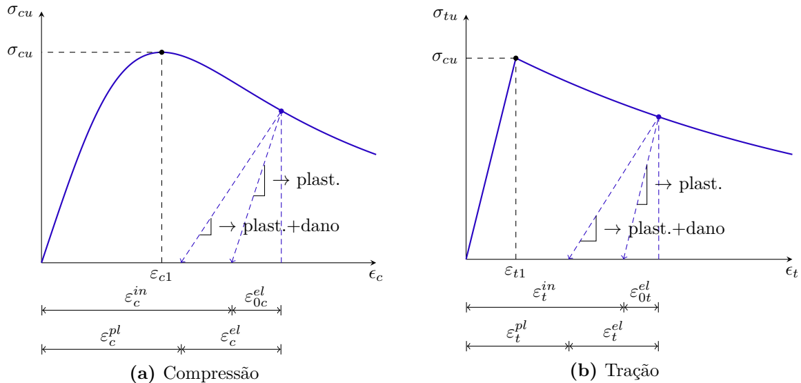
Figura 3.23 – Relação tensão-deformação no CDP
